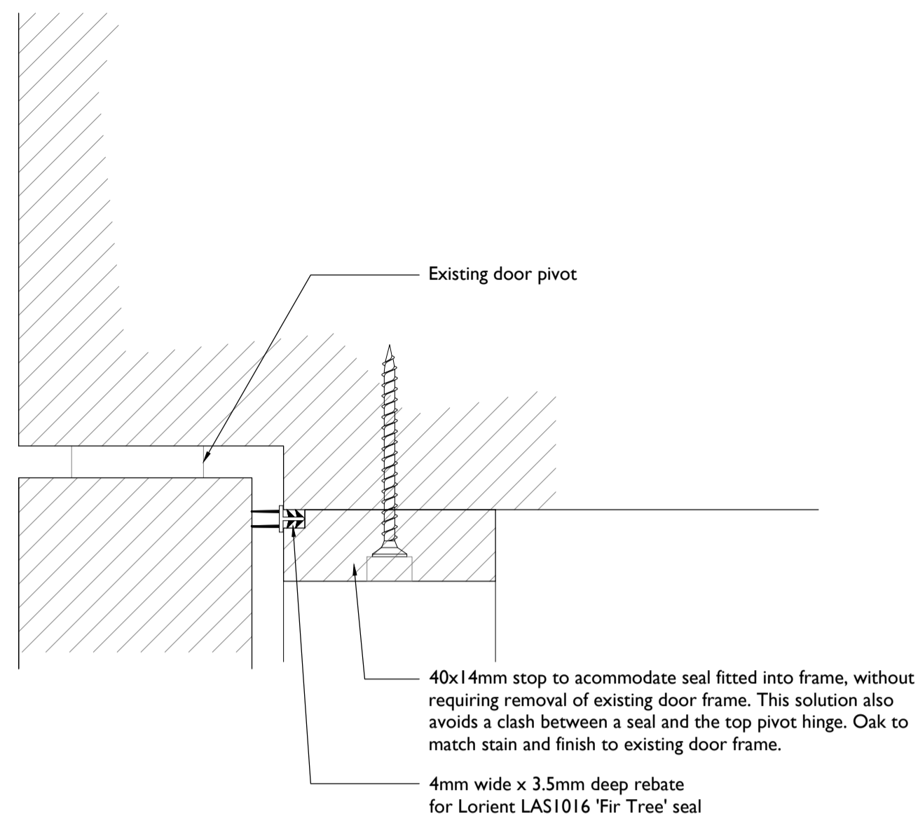
1 DOOR HEAD DETAIL 1:1
