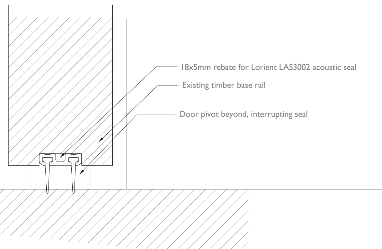
5 DOOR BASE DETAIL 1:1
