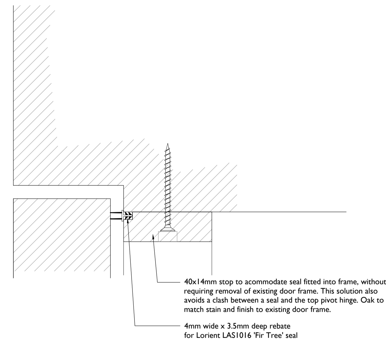
2 DOOR JAMB DETAIL 1:1
