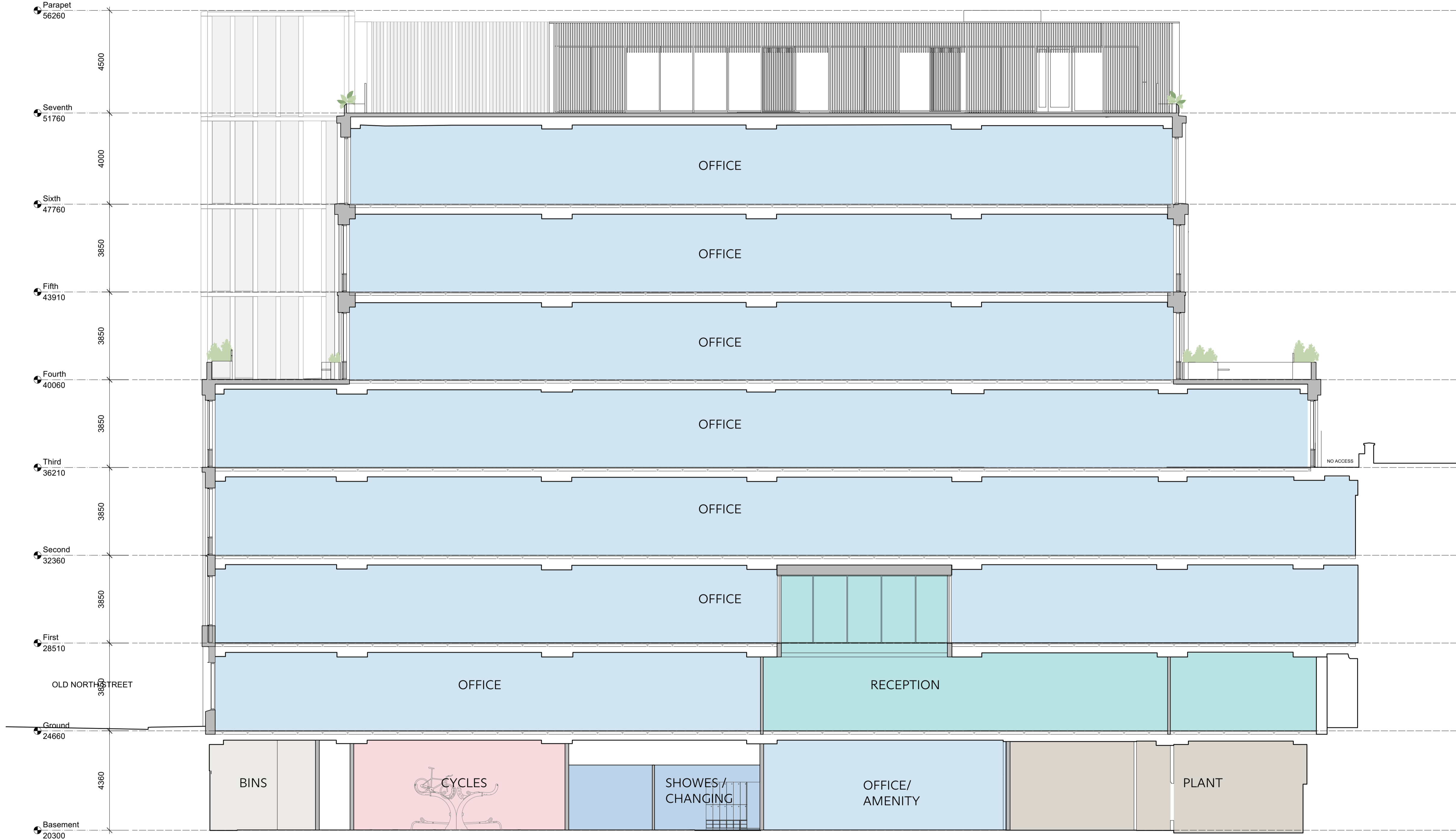
1 Section EE Scale: 1:100
