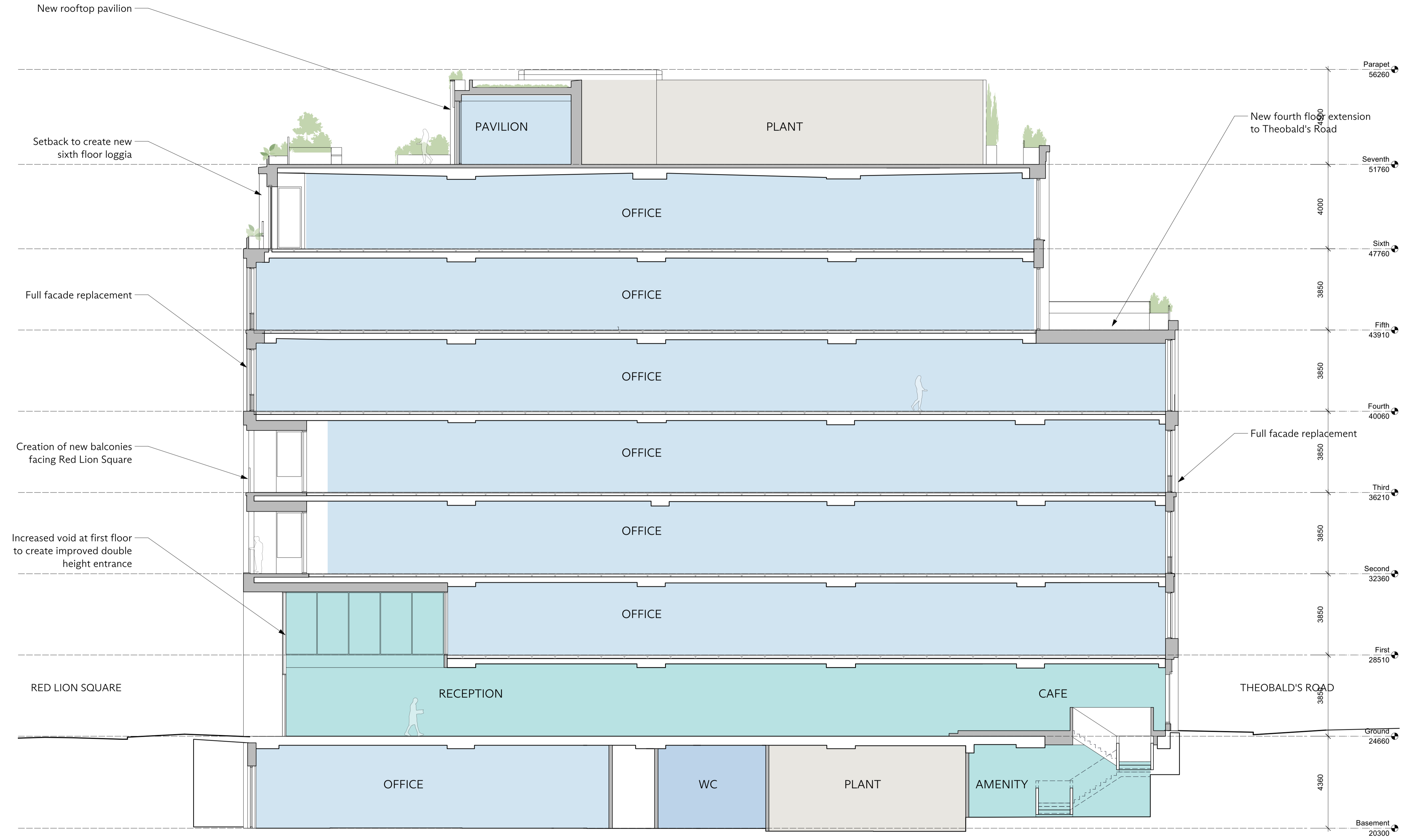
1 Section BB Scale: 1:100
