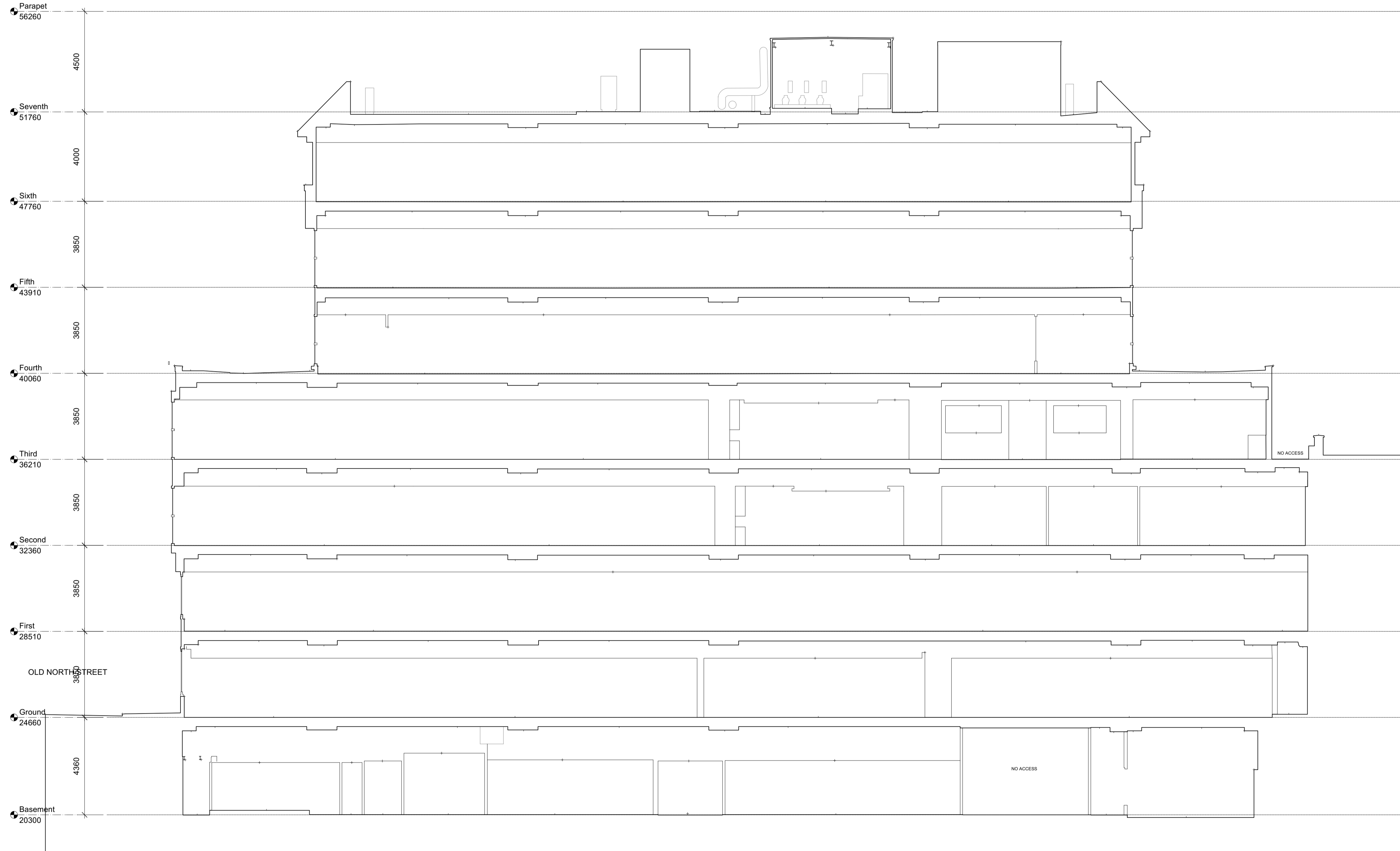
1 Existing Section EE Scale: 1:100
