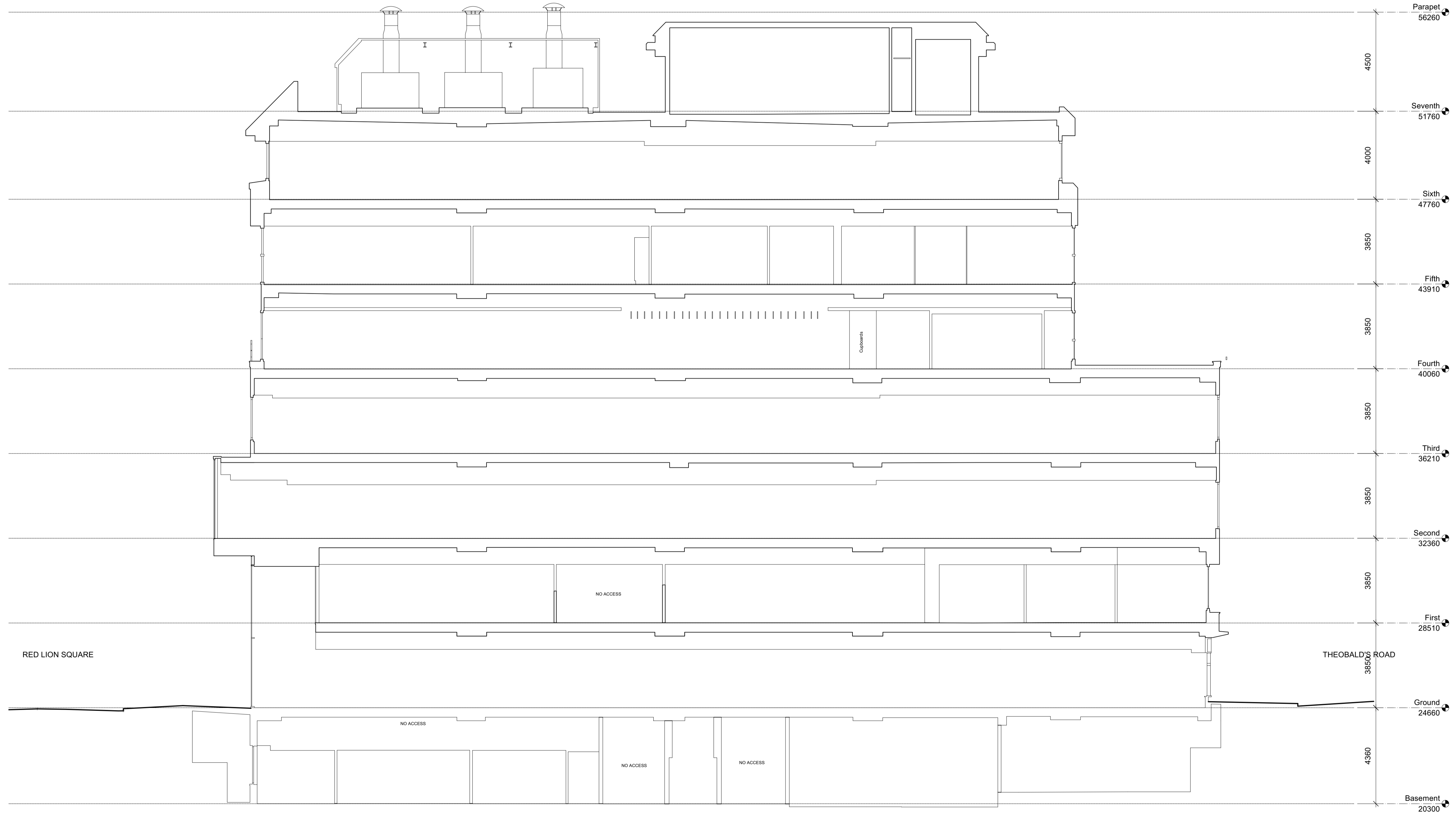
1 Existing Section BB Scale: 1:100
