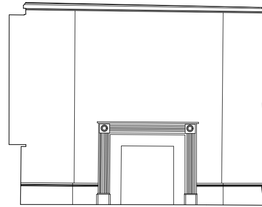
Elevation 1
