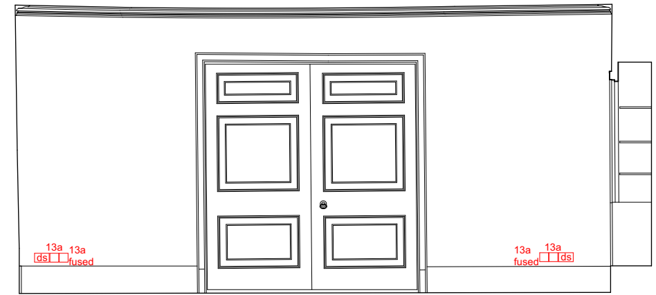
Elevation 4
