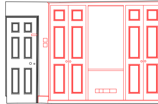
Elevation 2
