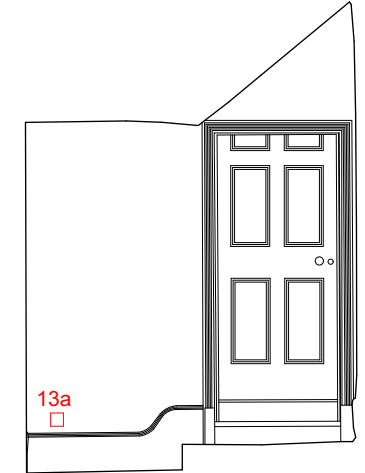
Elevation 4
