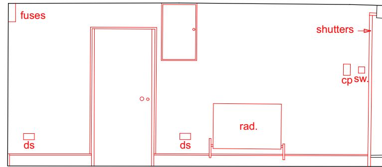
Elevation 1
