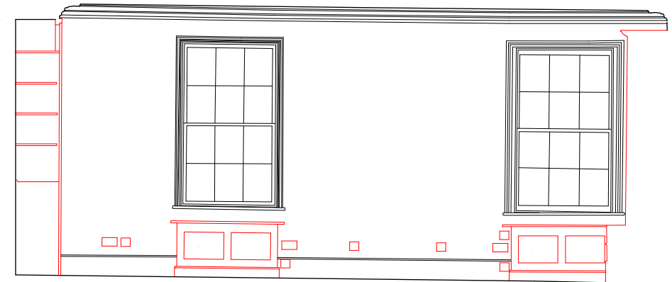
Elevation 2
