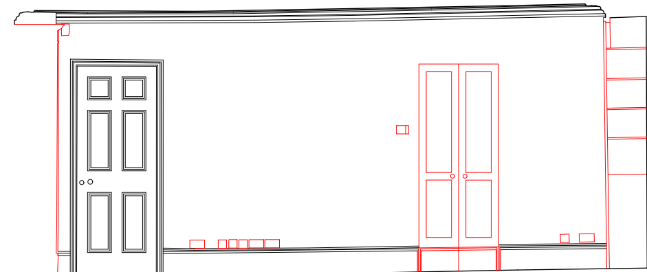
Elevation 4
