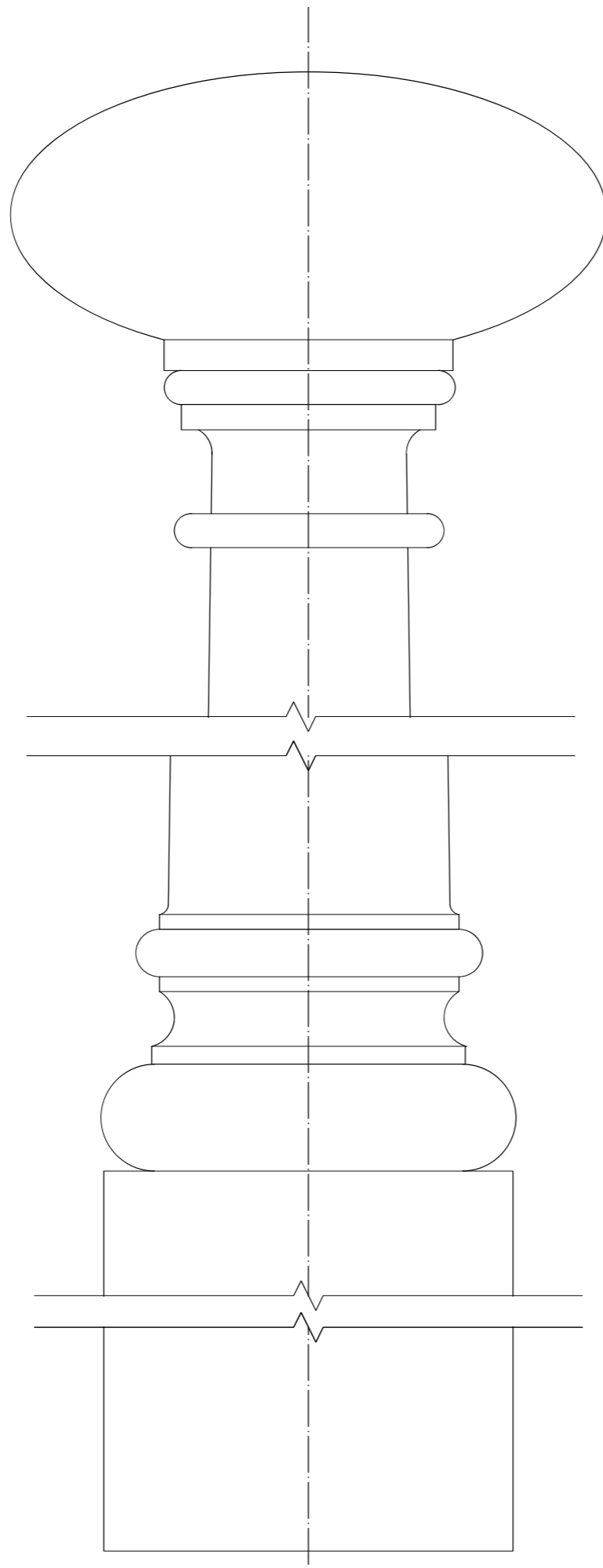
2 Newel detail (24)02 Scale: 1:1@A3
