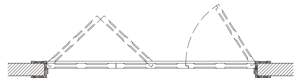
1 Timber Door - Plan 1:20
