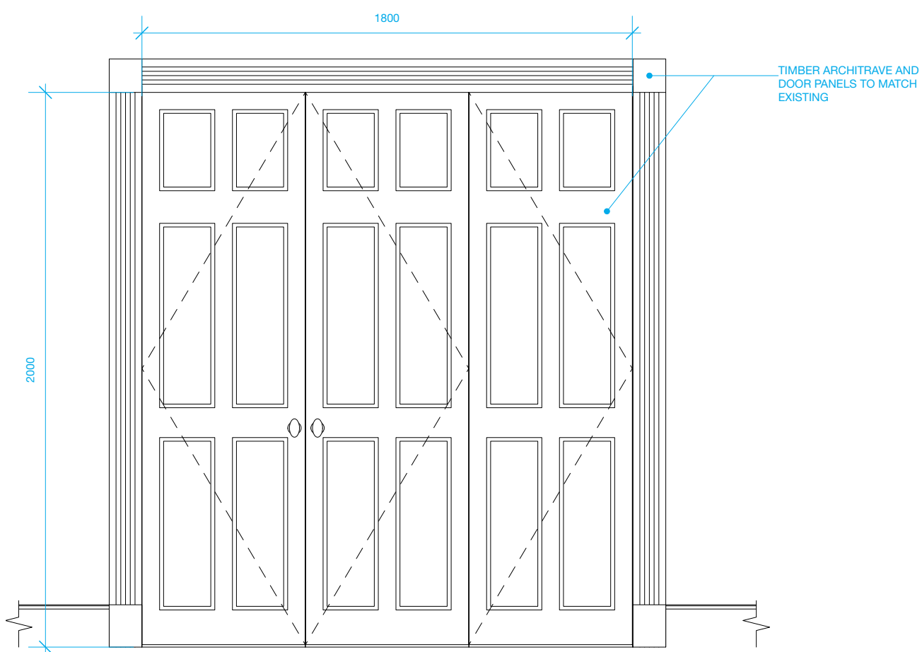
2 Timber Door - Elevation 1:20
