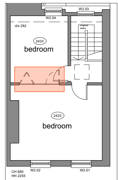
2F internal Door Plan - Bedroom 1:100
