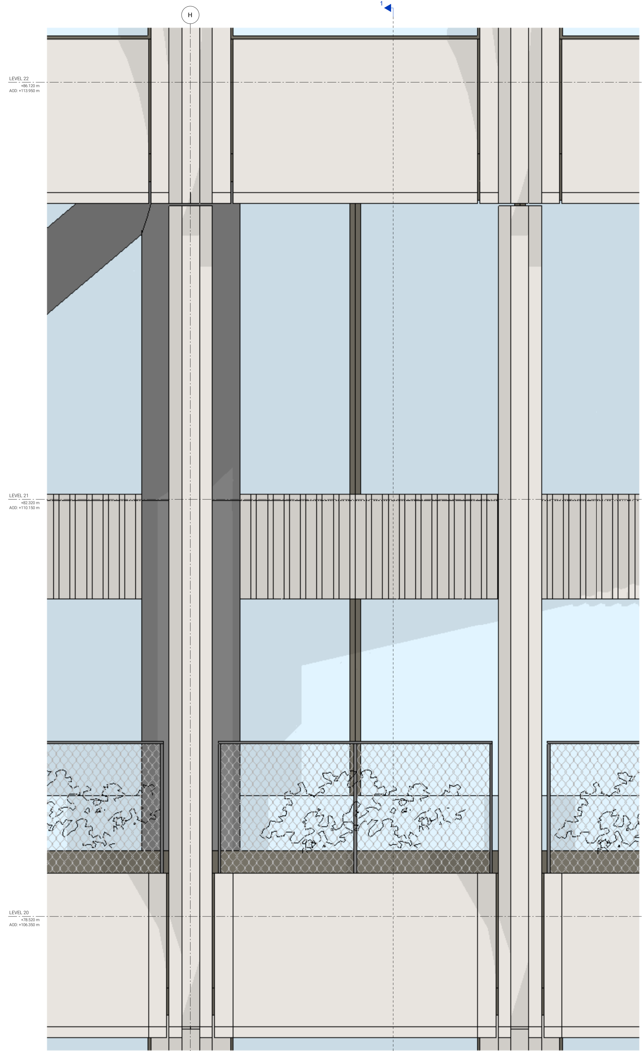
ELEVATION 1:20
