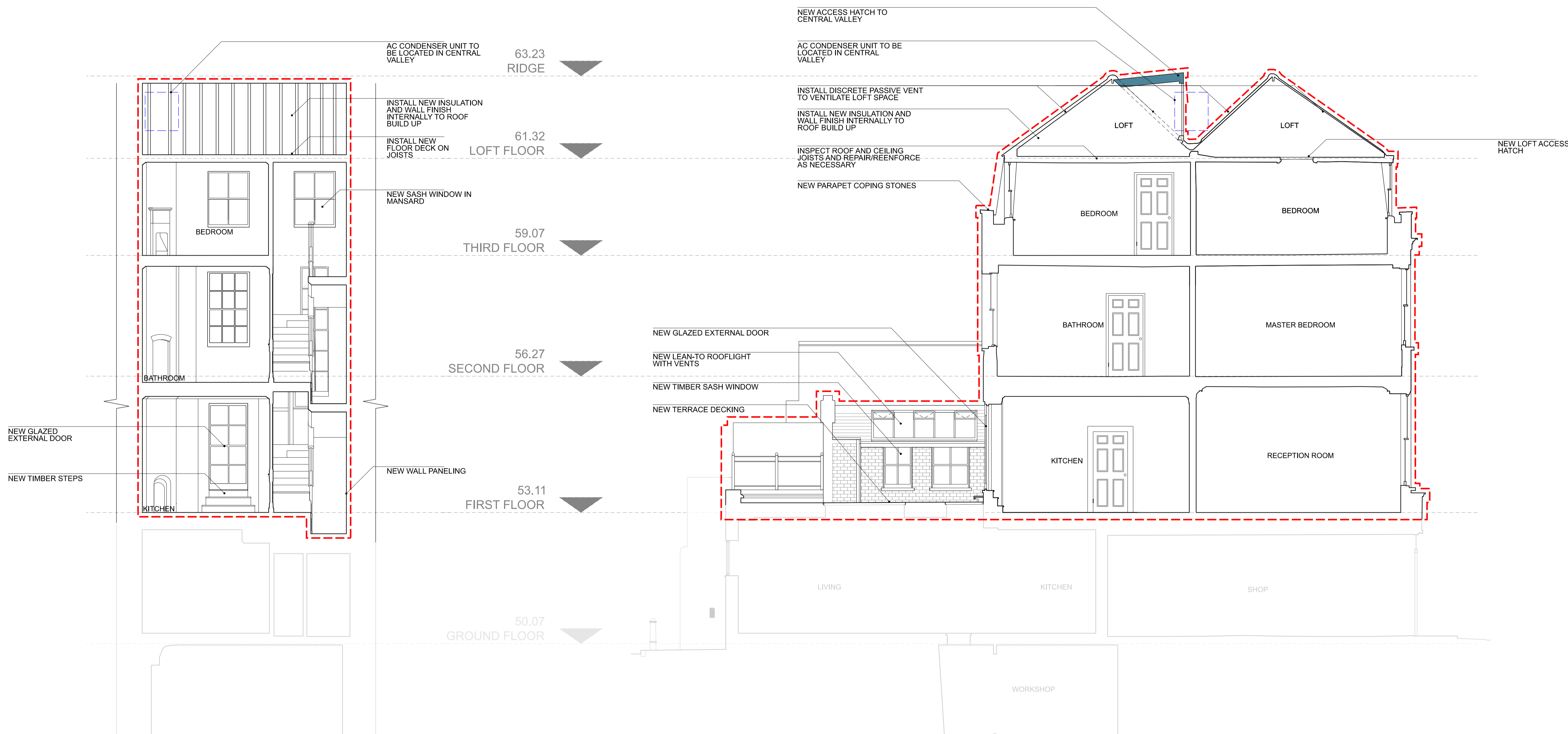
1 1:50 @ A1 | 1:100 @ A3 SECTION A
