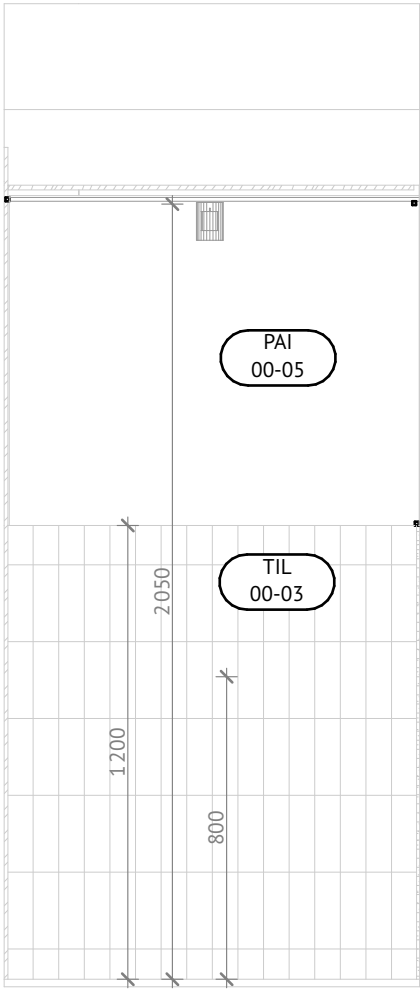
GF.02-02 GA-WC - 1:20
