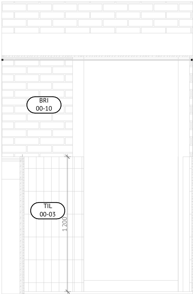
GF.02-01 GA-WC - 1:20
