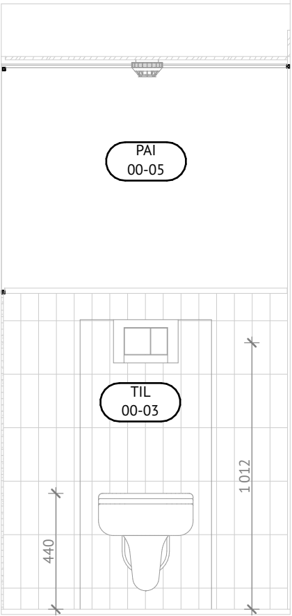
GF.02-04 GA-WC - 1:20
