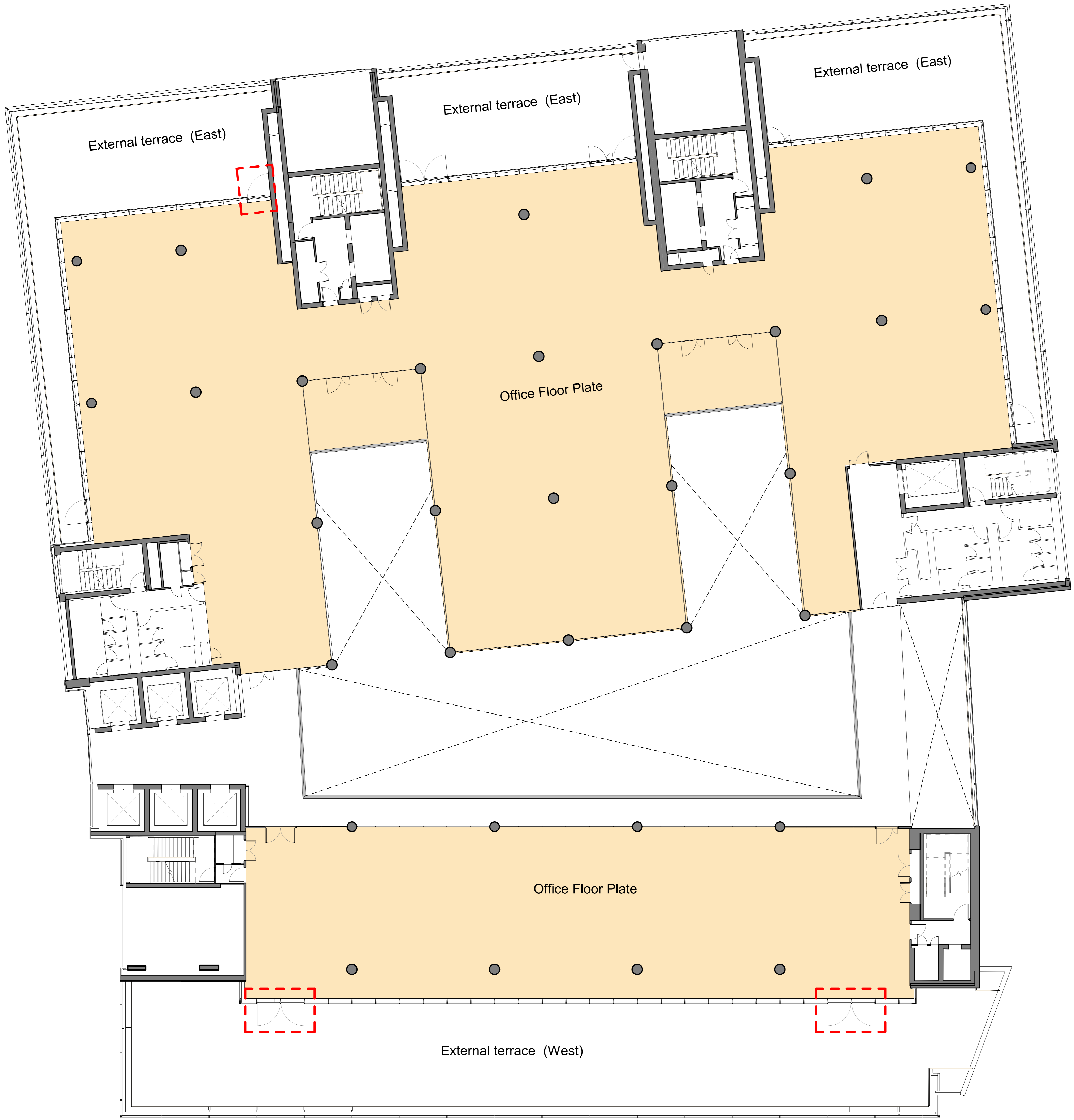
1 Existing L06 Plan 1 : 100
