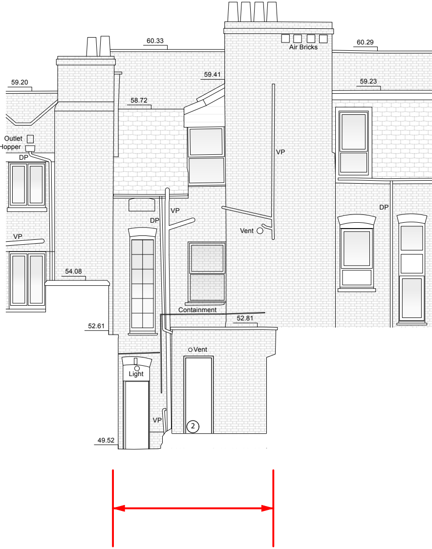
ELEVATION 2
