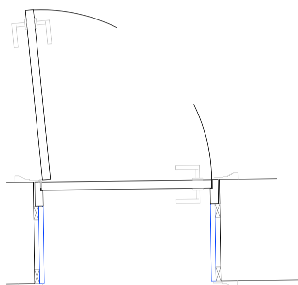
DG-03 / DG-06 Solid 4 panels timber door
