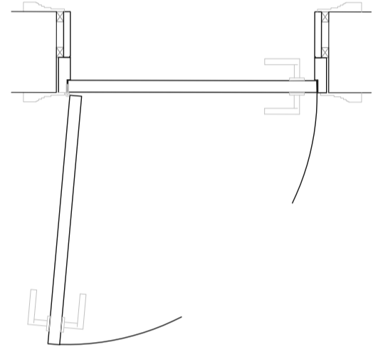
DG-04 Solid 4 panels timber door
