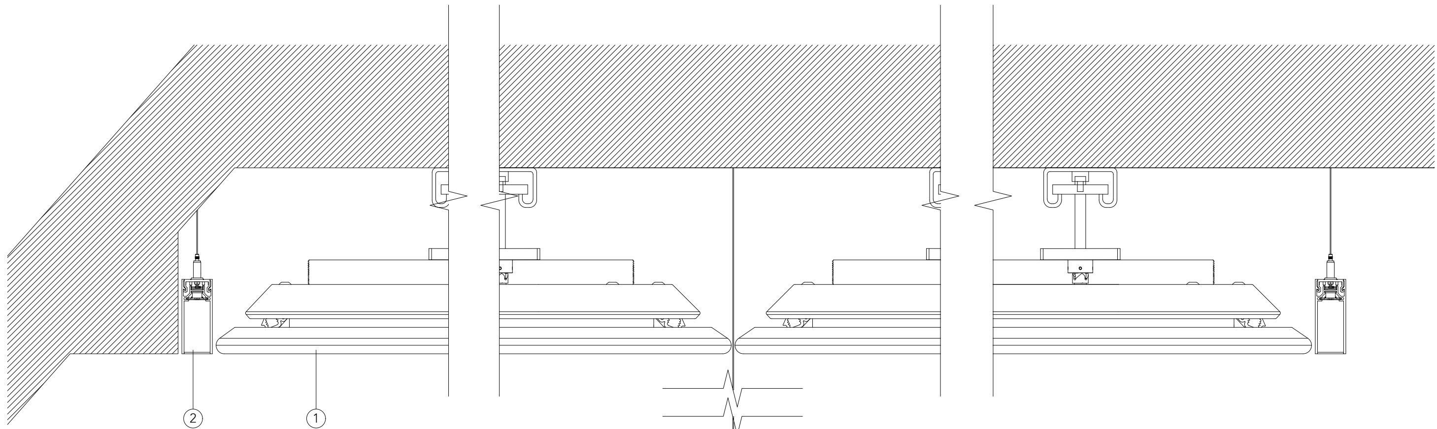
1 Ceiling raft - long section Scale: 1:5
