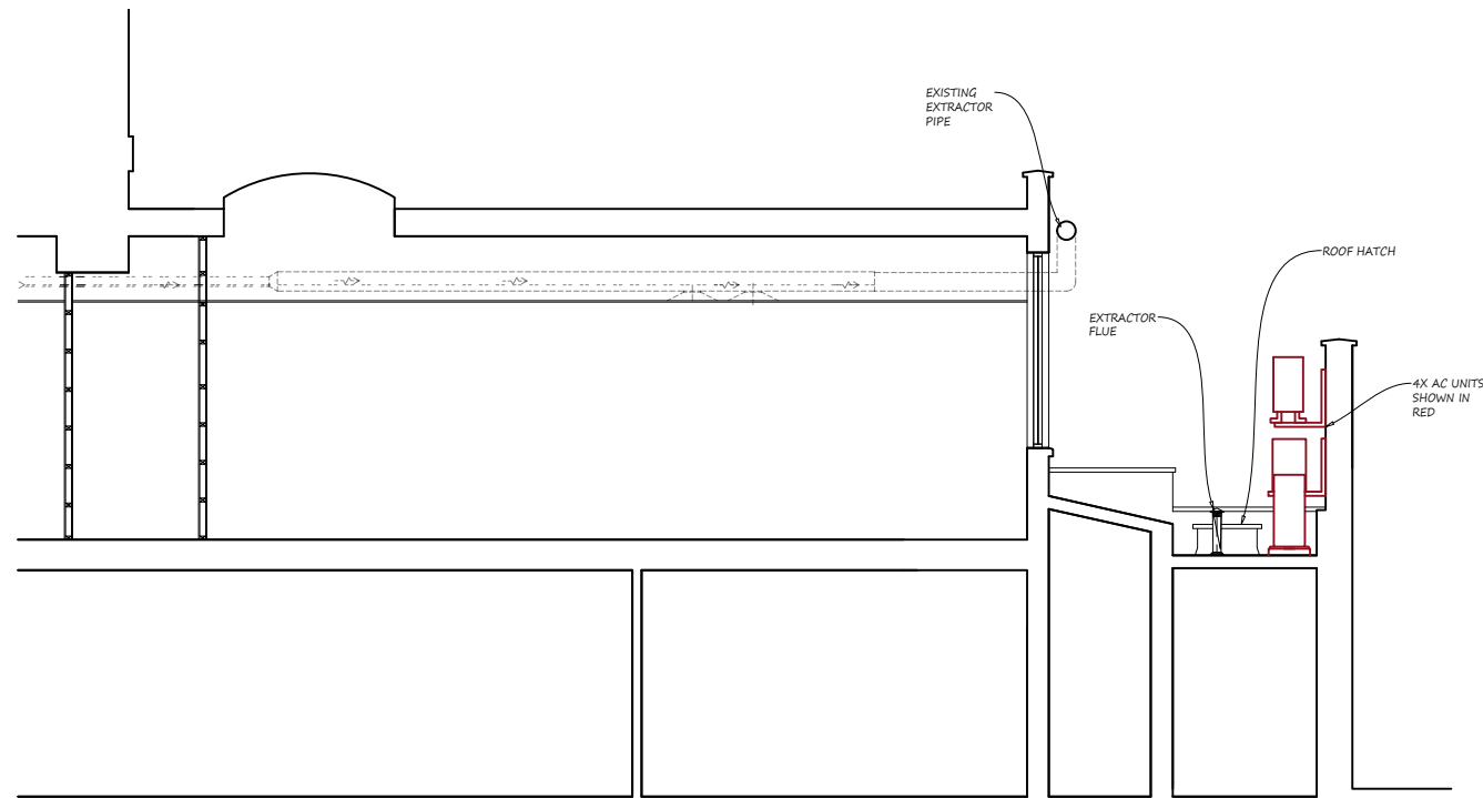
EXISTING SECTION A-A 1:100
