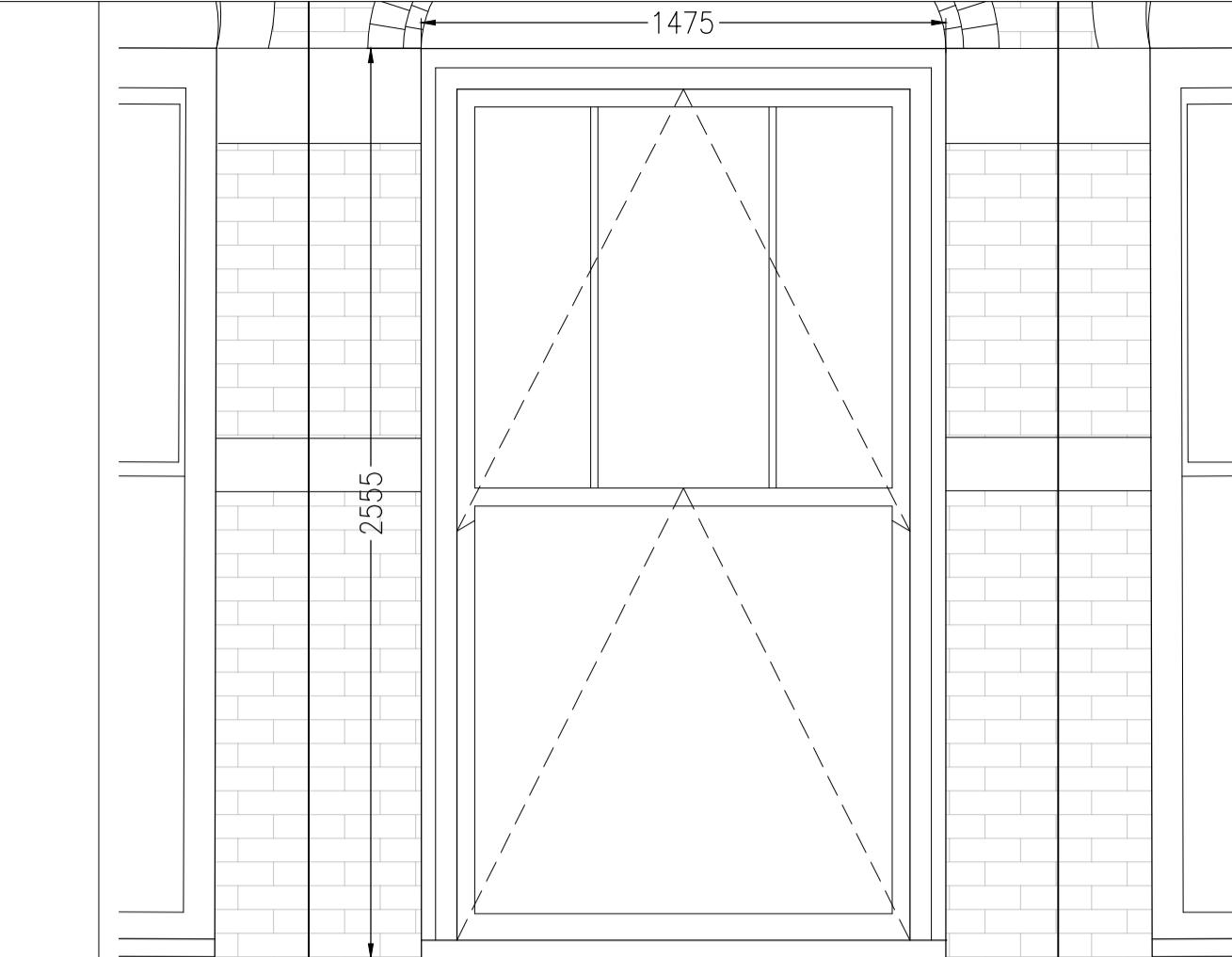
WINDOW TYPE 'B' 1:20
