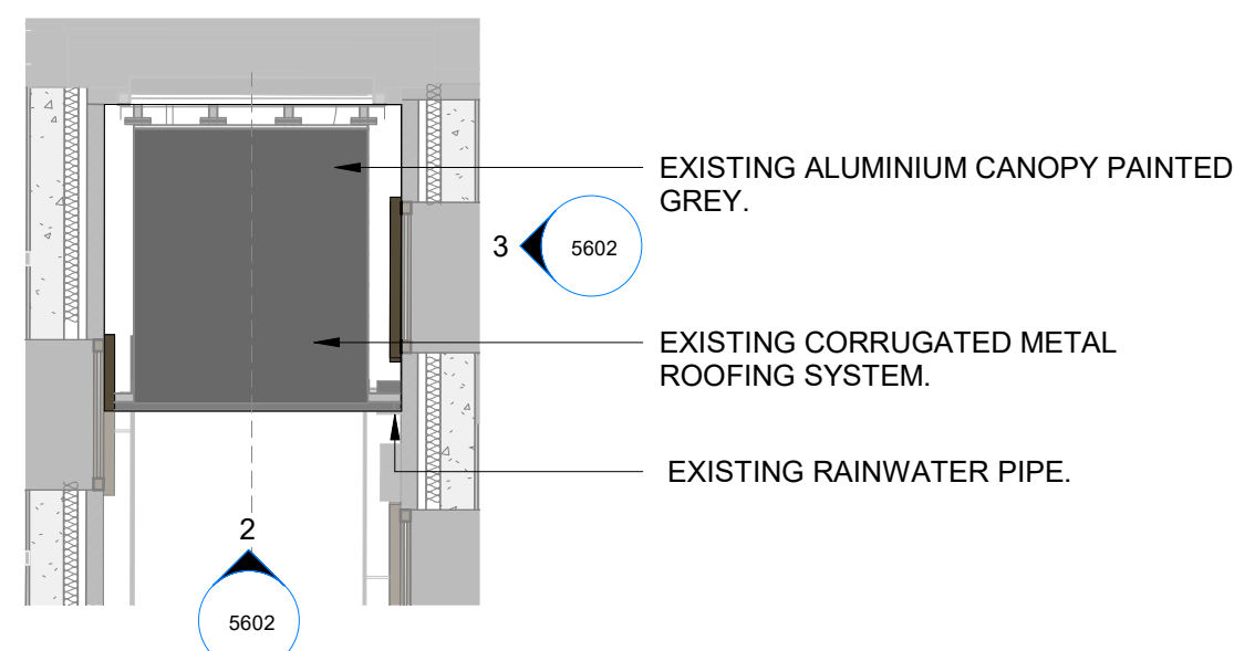
7 T4 - CANOPY 01 - EXISTING PLAN 1 : 50
