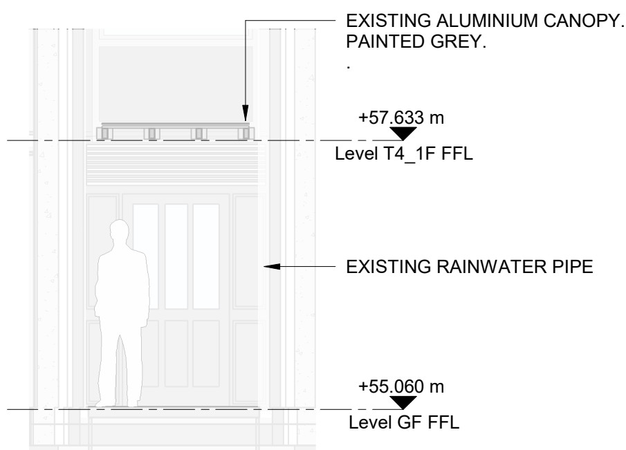
6 T4 - CANOPY 1 - EXISTING SECTION 3 1 : 50
