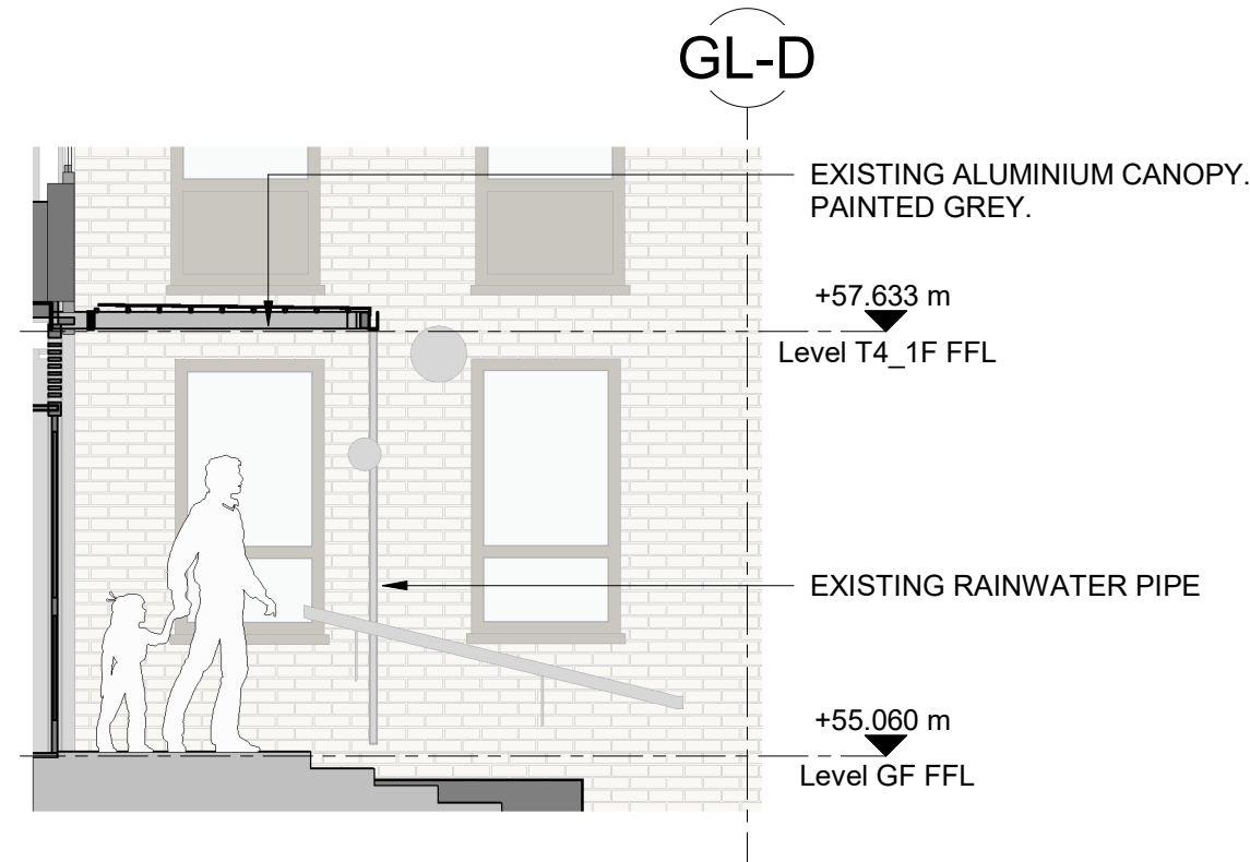
4 T4 - CANOPY 1 - EXISTING SECTION 1 1 : 50
