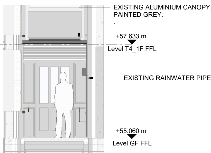
5 T4 - CANOPY 1 - EXISTING SECTION 2 1 : 50
