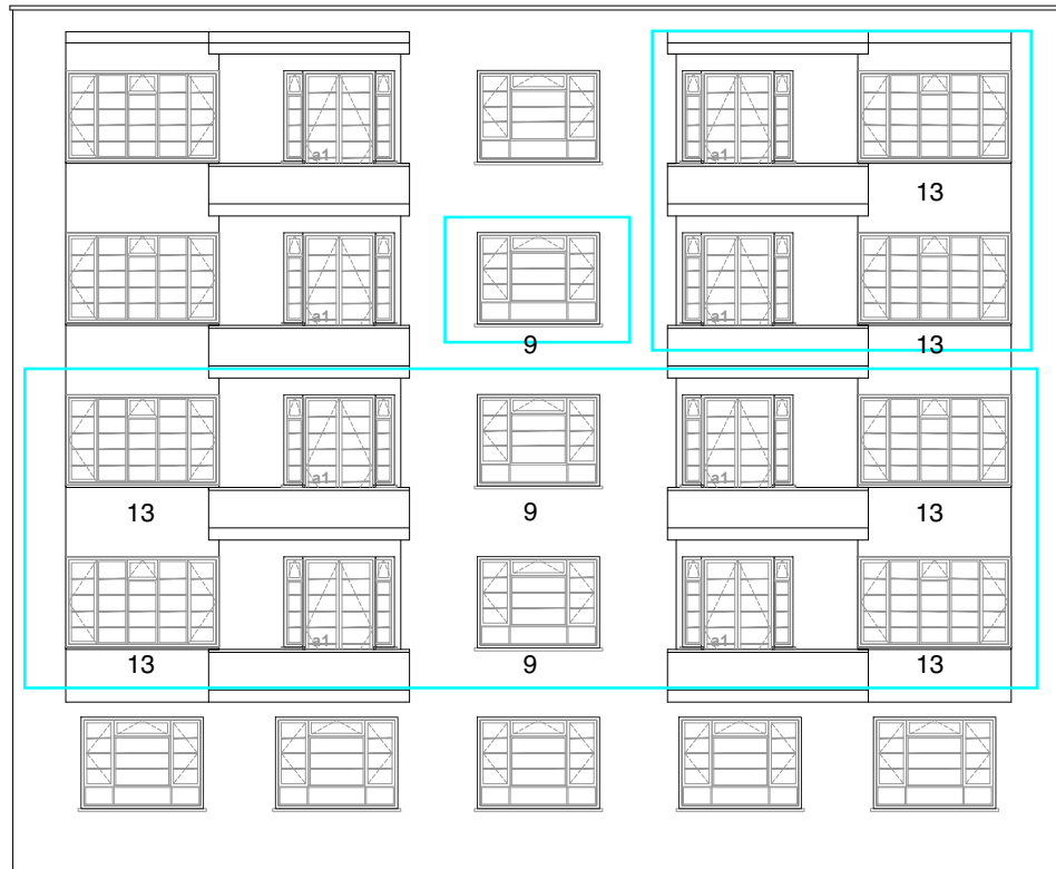
ELEVATION J
