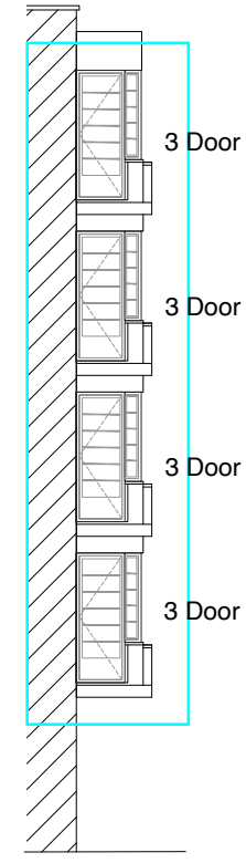
ELEVATION L
