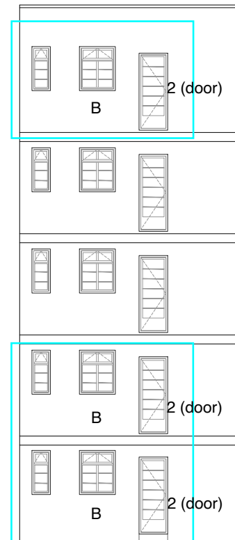
ELEVATION T
