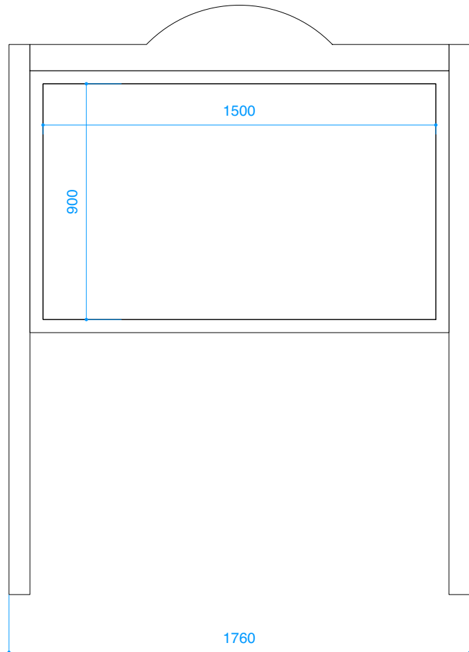
ELEVATION
