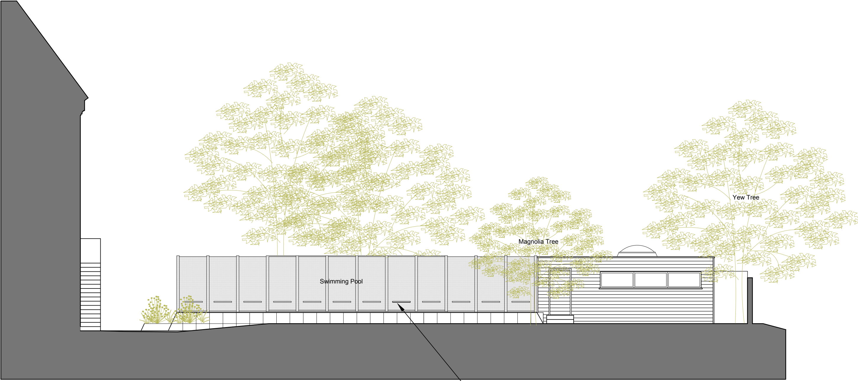
Existing Elevation D:D
