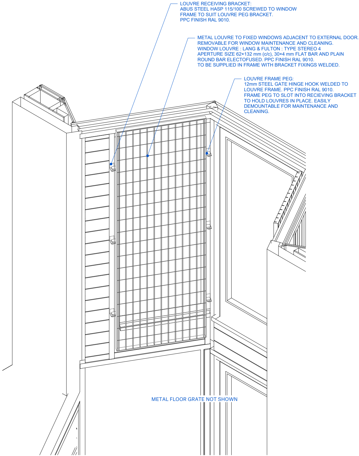
2 AXO VIEW : WINDOW GRATE Scale: 1:20
