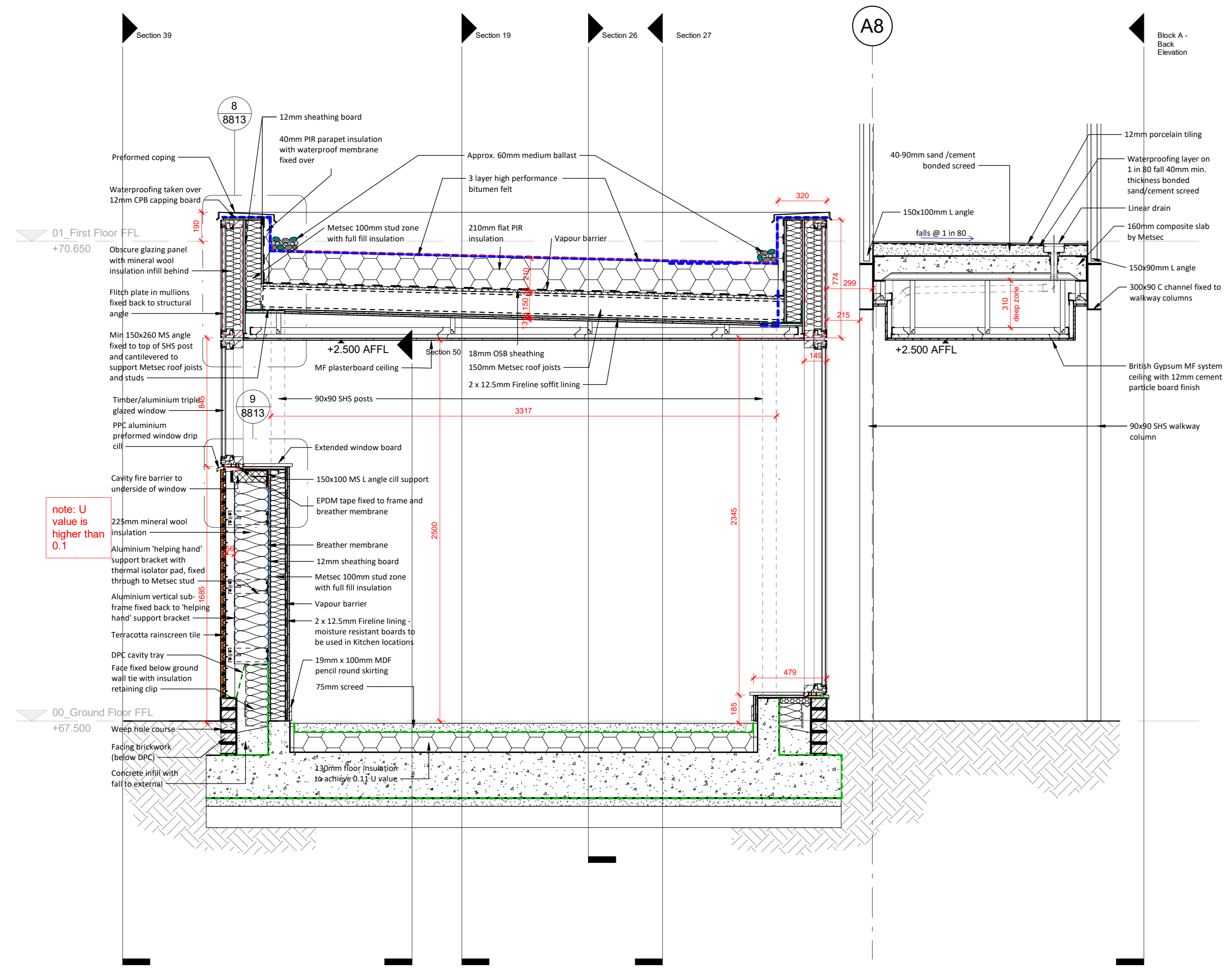
1 Section 25 1 : 20
