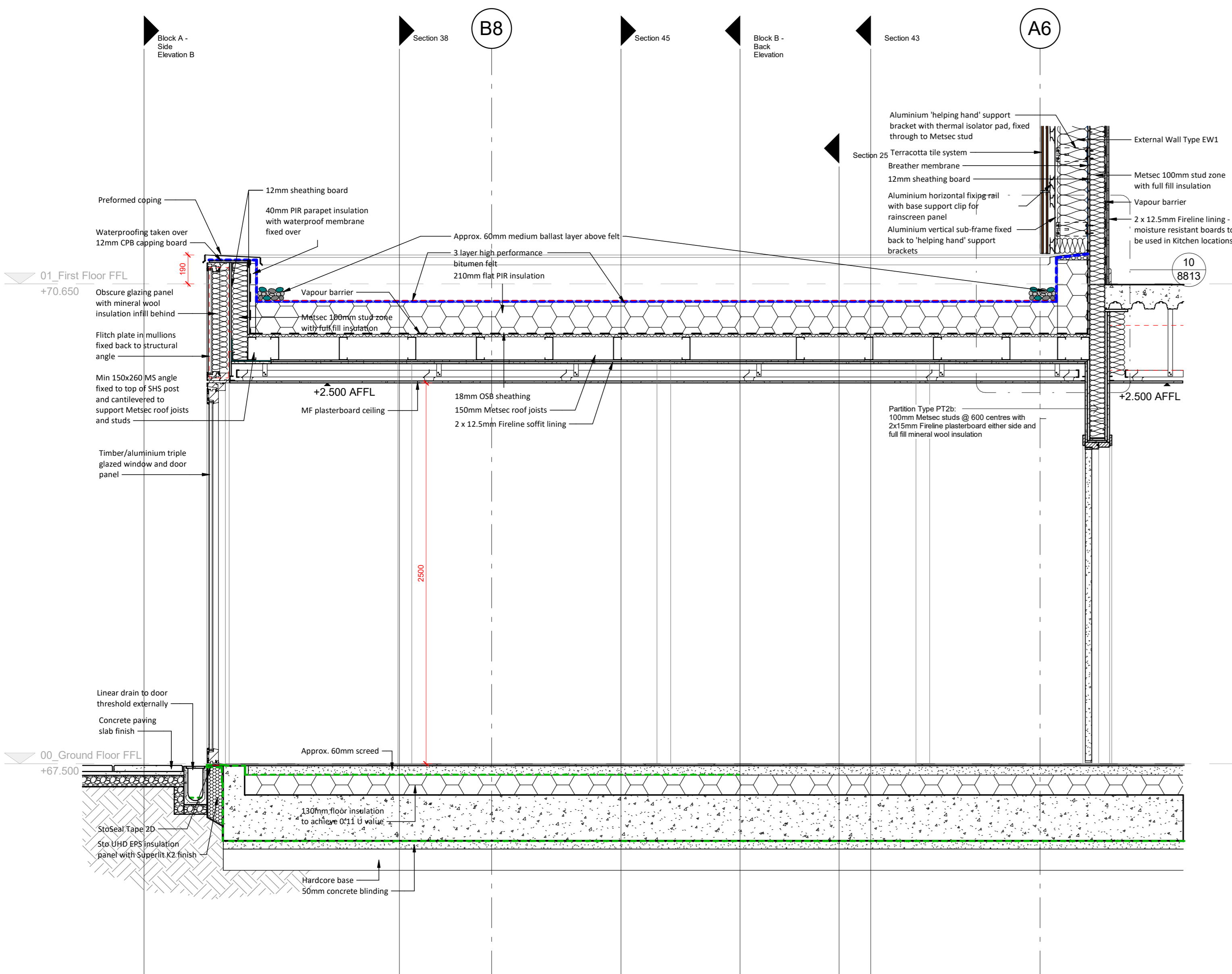
2 Section 26 1 : 20
