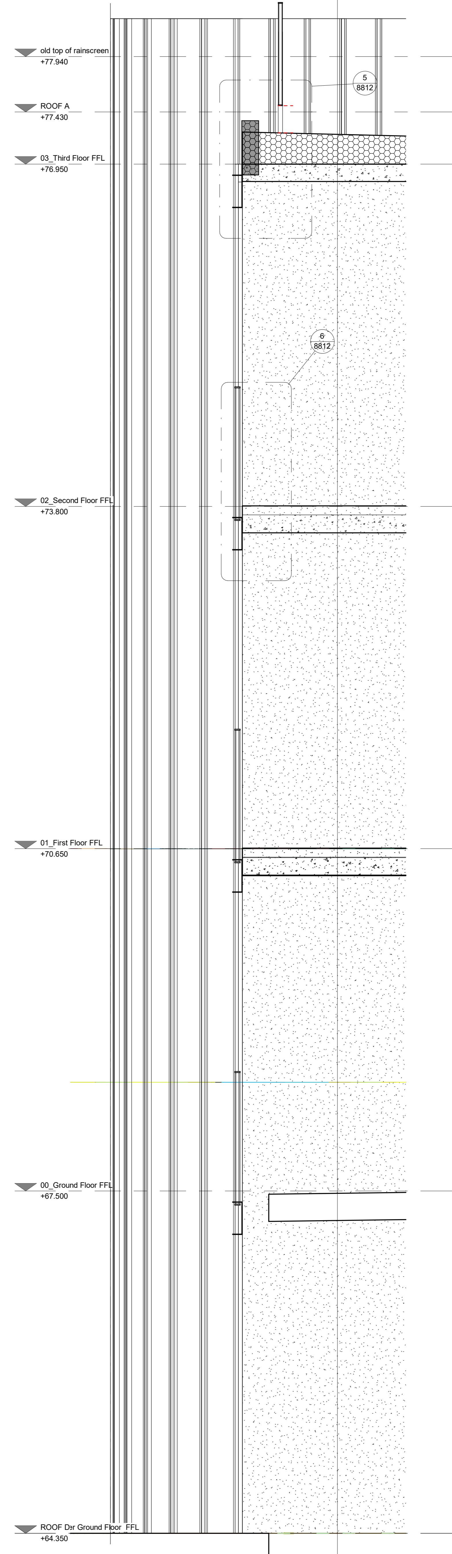
3 Section 28 1 : 20
