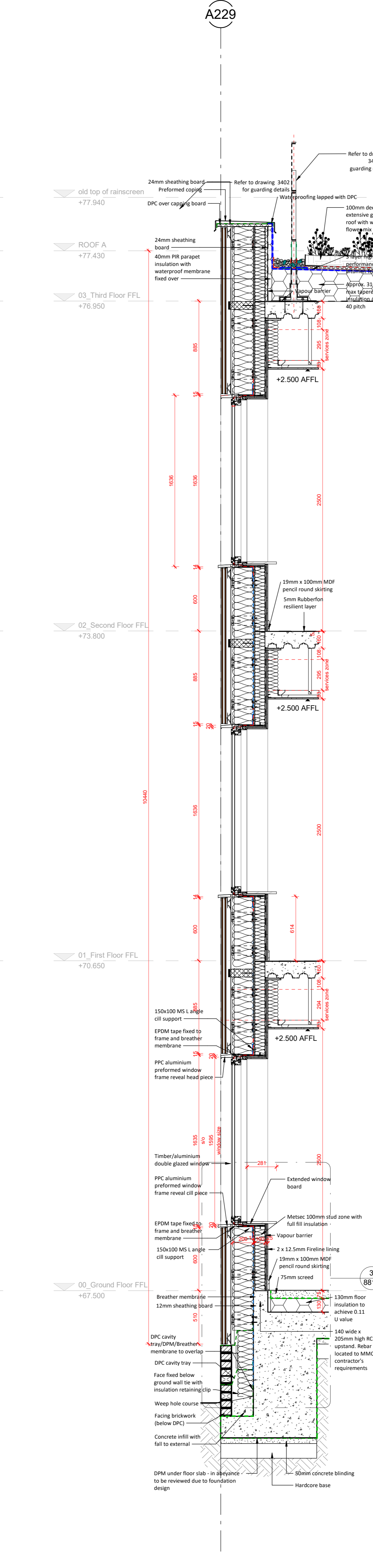
3 Section 5 - Callout 1 1 : 20
