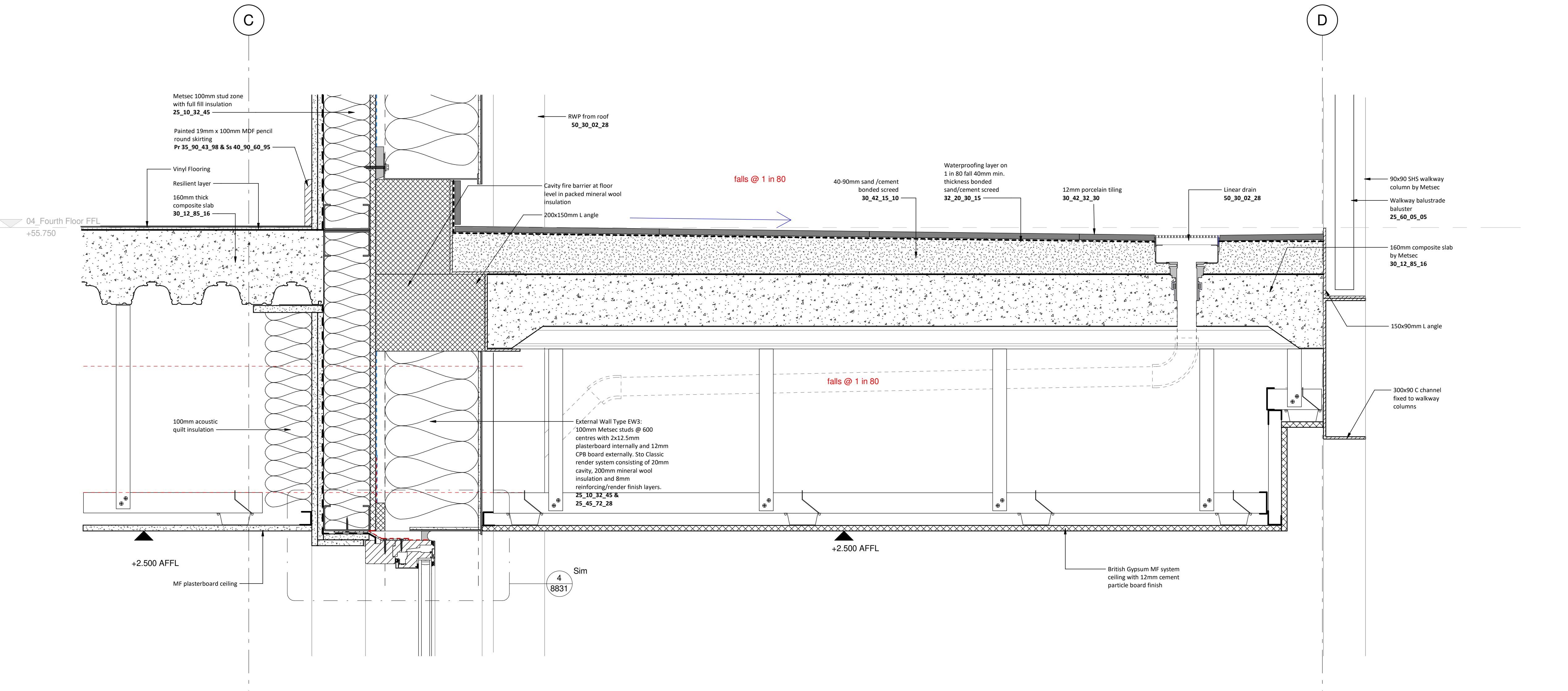
4 Section 1 - Callout 2 - Callout 2 1 : 5
