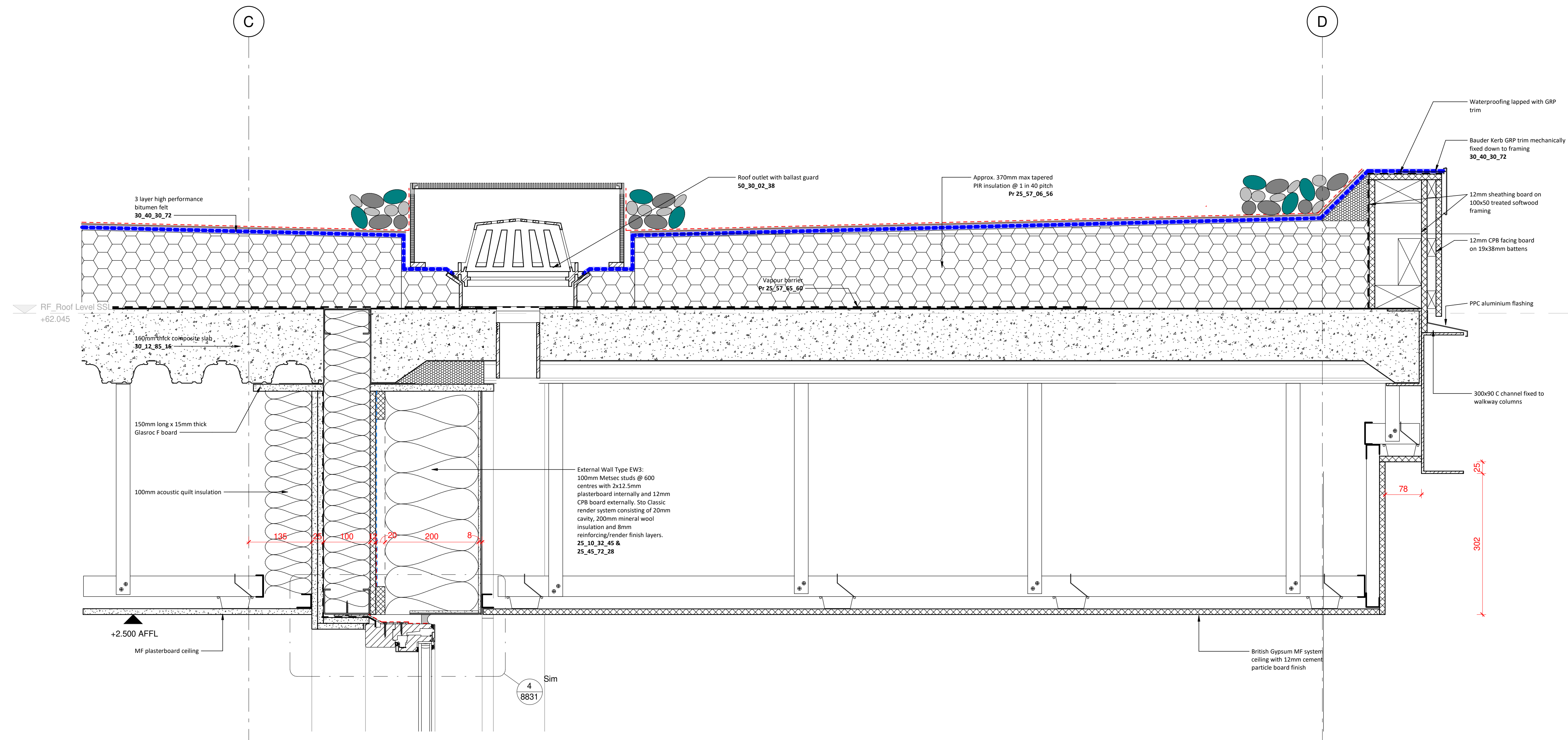
3 Section 1 - Callout 2 - Callout 1 1 : 5
