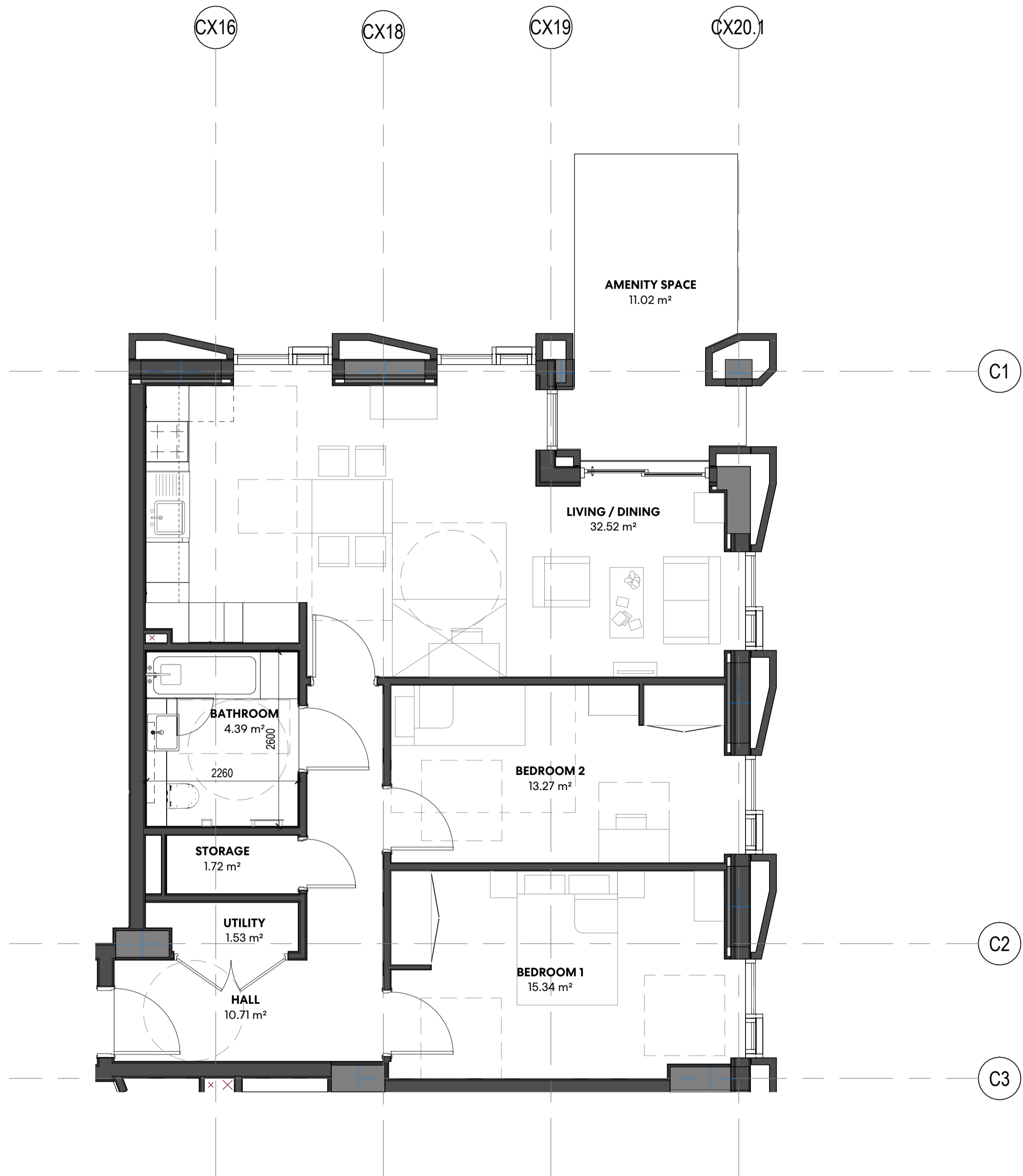
1 FLAT TYPE P.2b-D (WA) Planning 1 : 50
