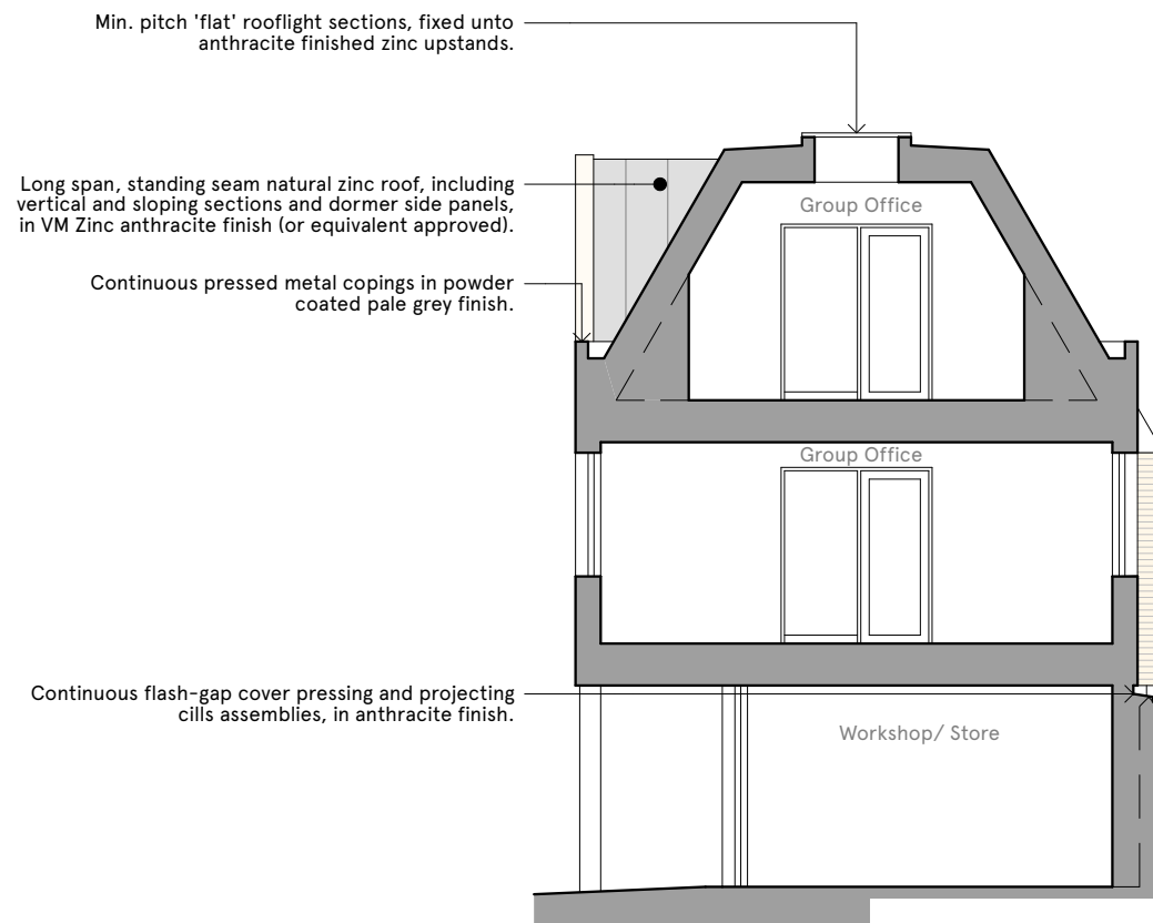
Section A-A
