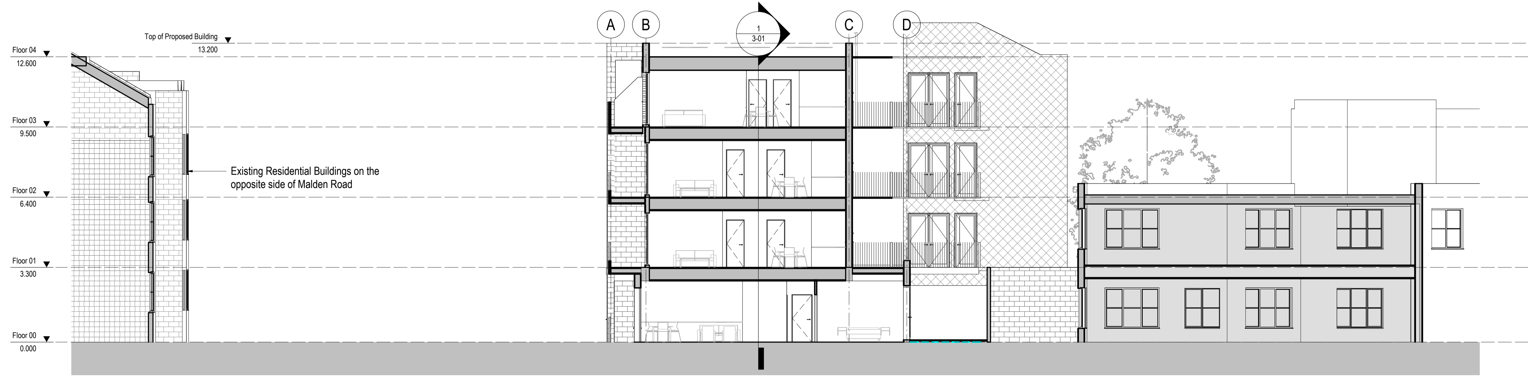
3 Section 3 1:100
