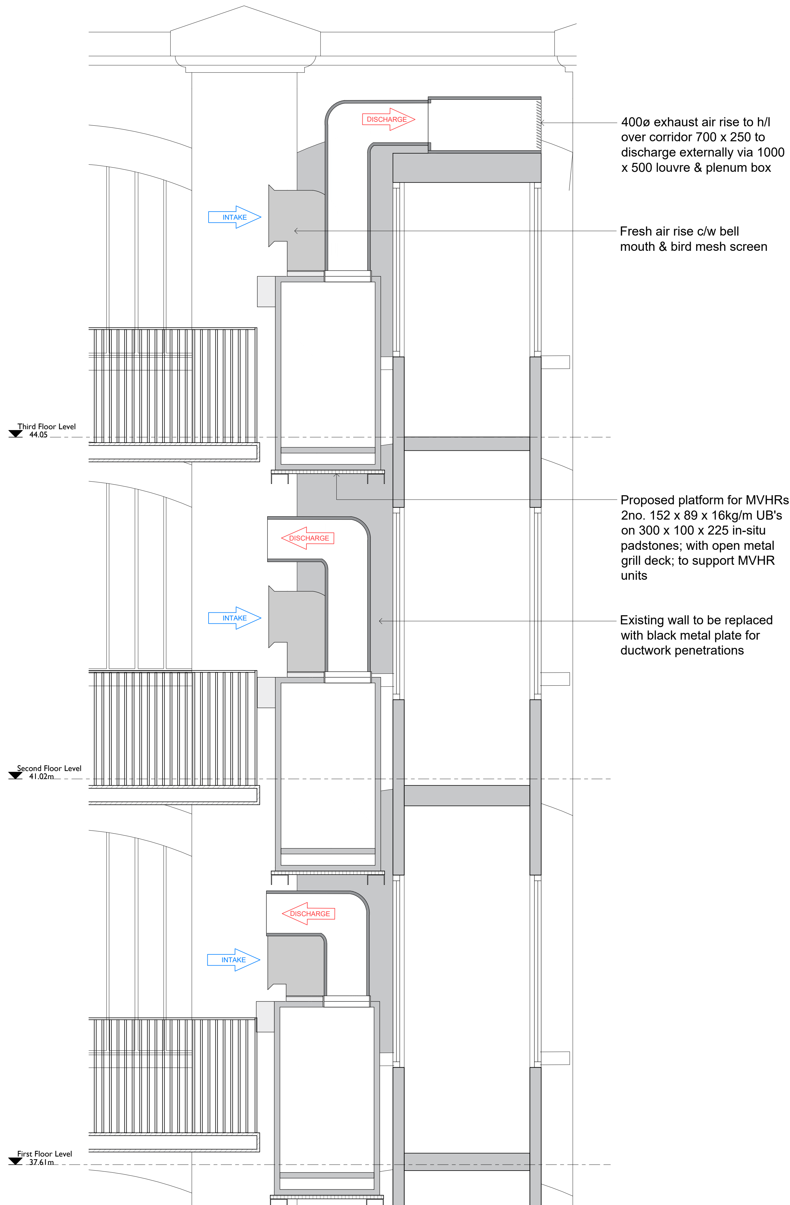
02 Section 480 1:20
