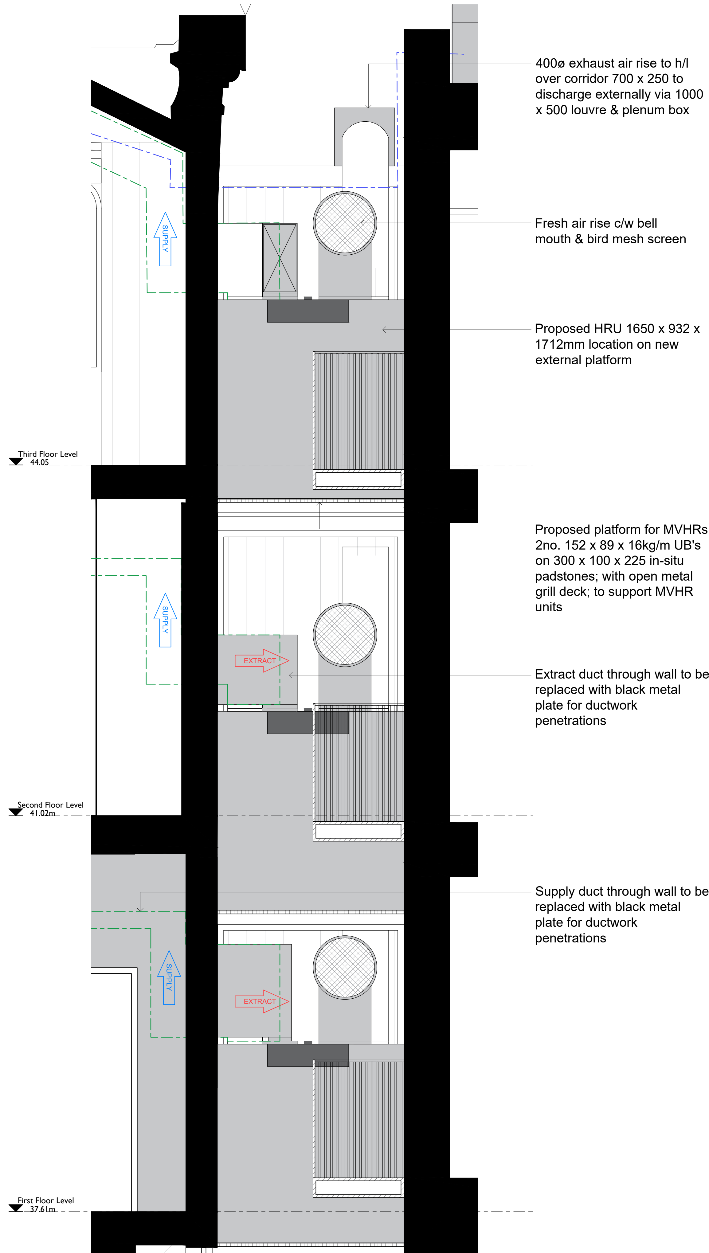
01 Elevation 480 1:20
