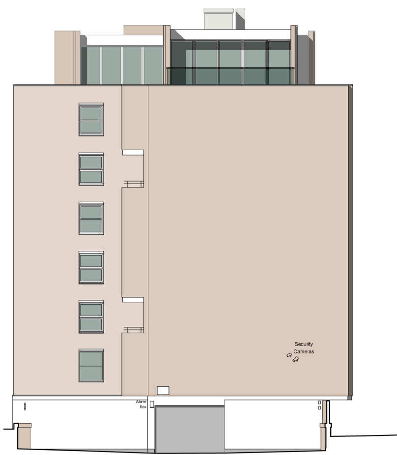
Elevation 2
