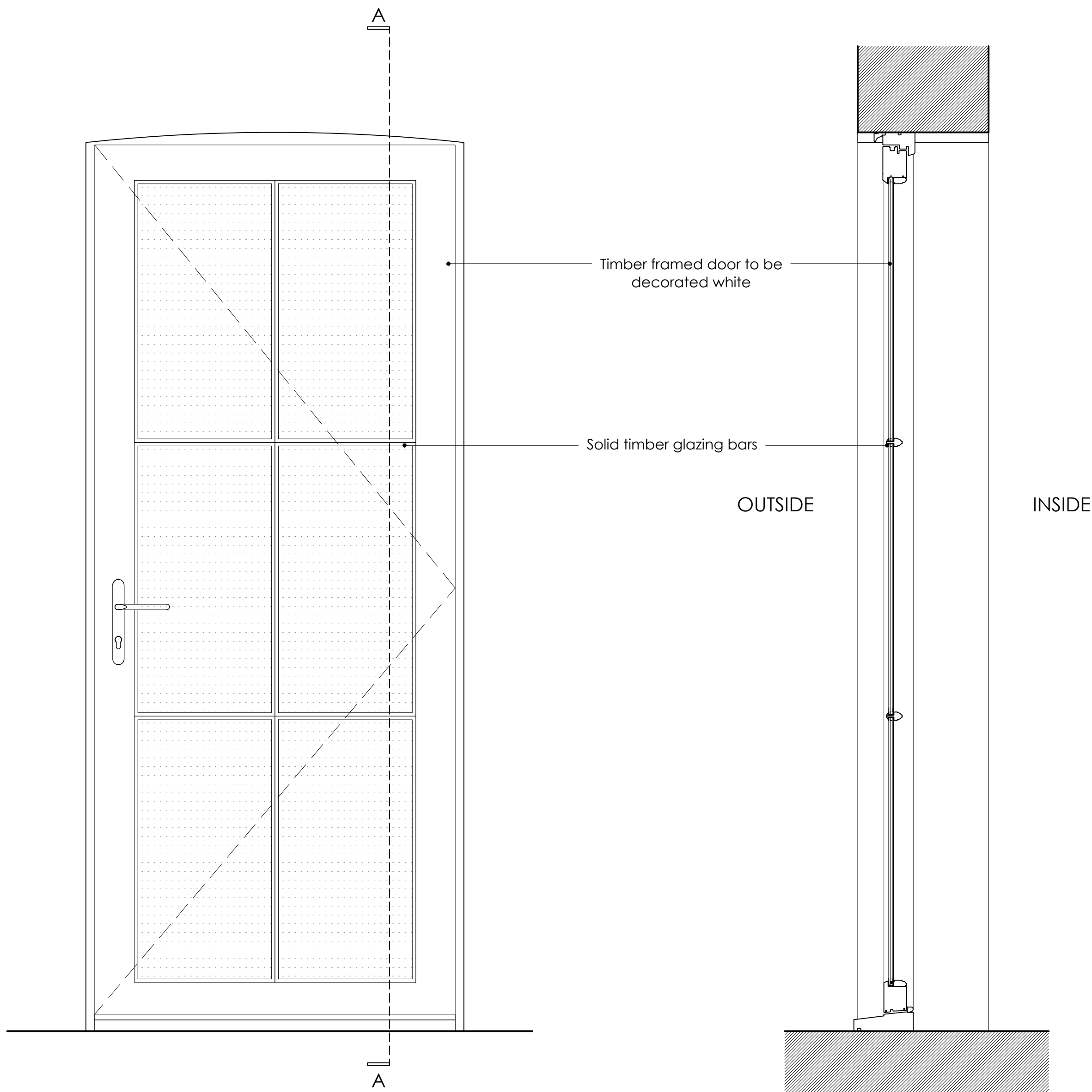
Door 1 Section AA
