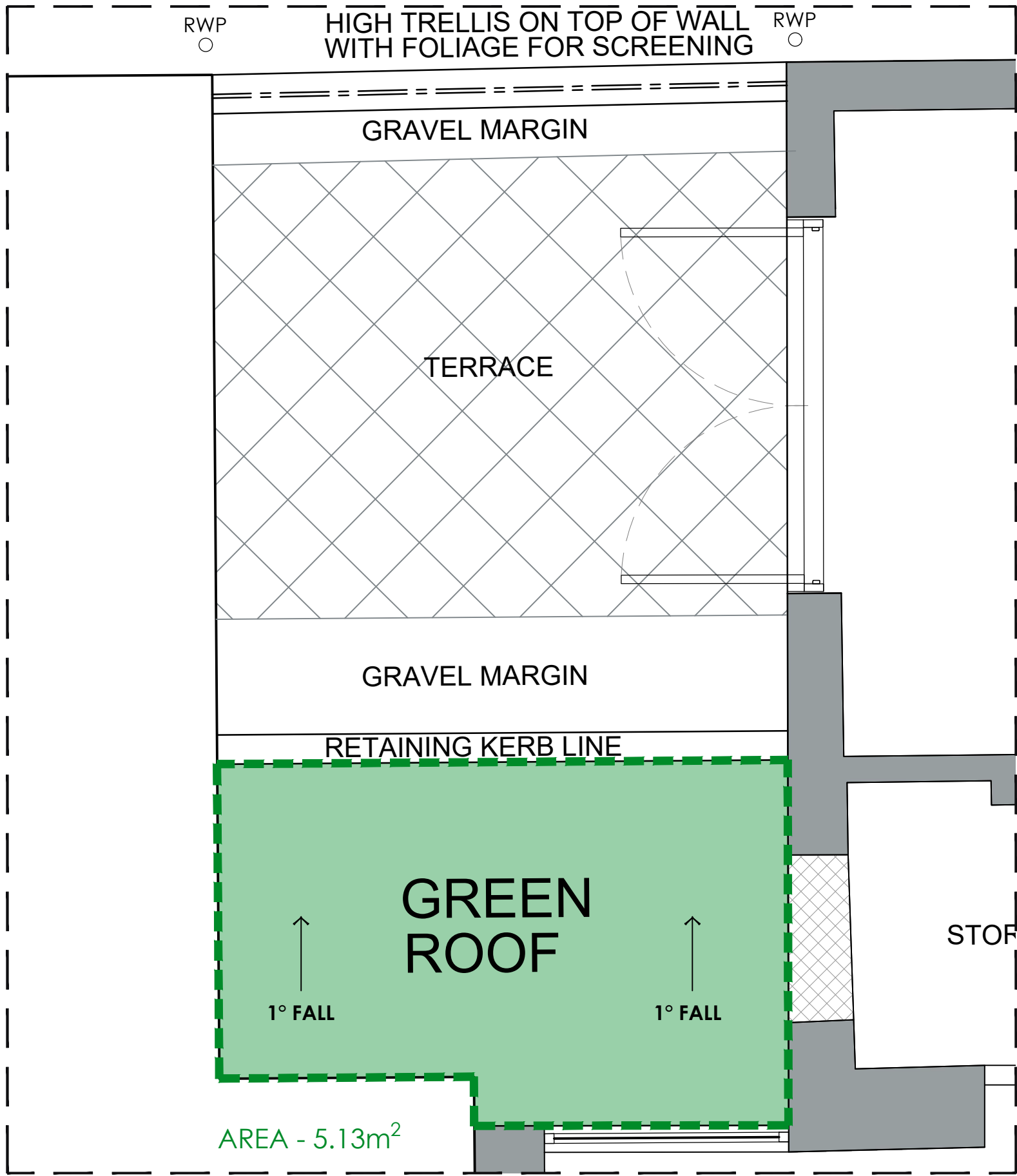
2 GREEN ROOF GA Scale: 1:20
