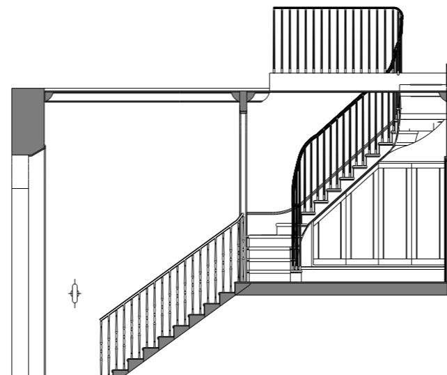
ELEVATION 01
