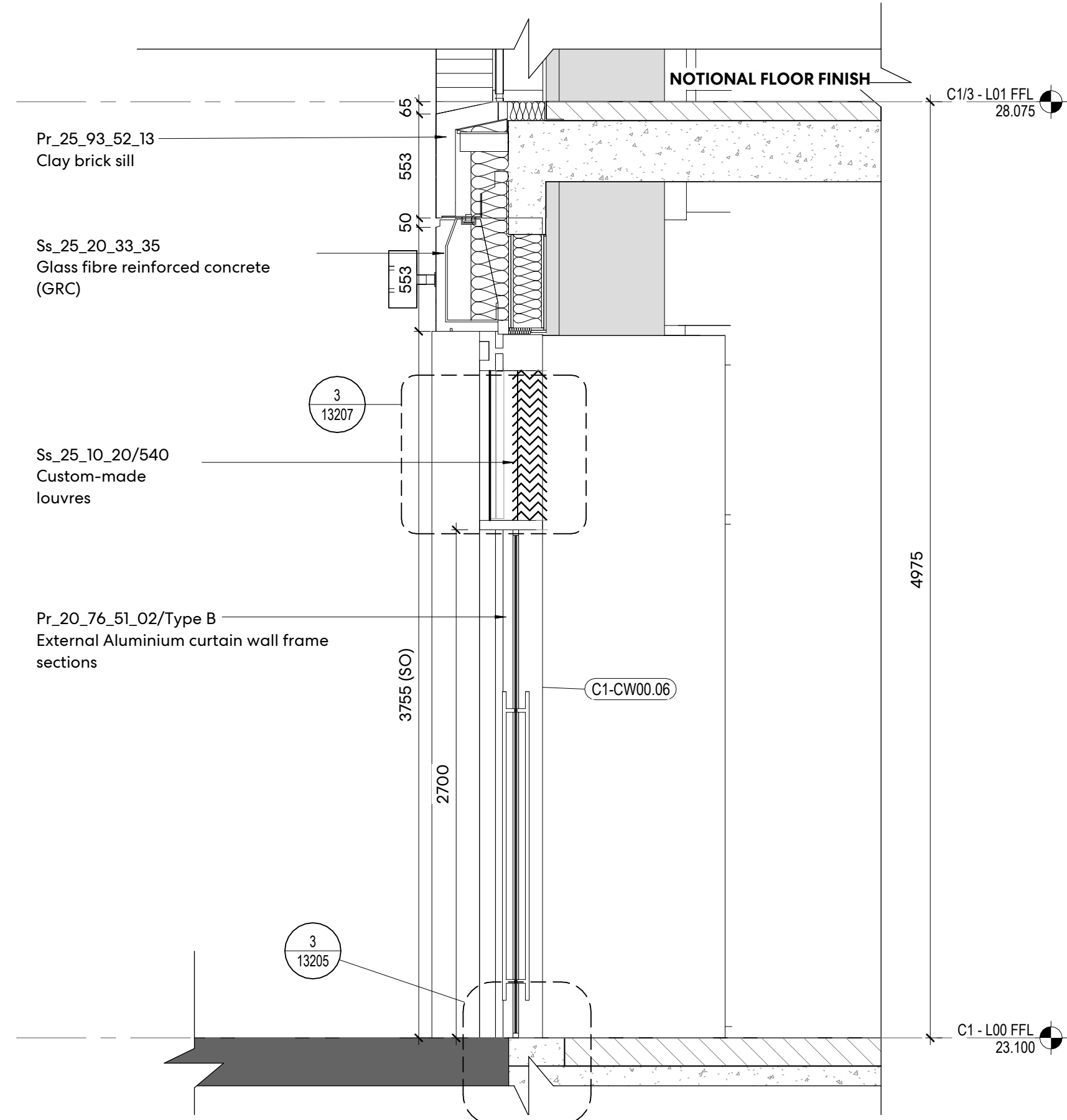
5 DOOR LEVEL 00-03 DETAIL SECTION 1:25
