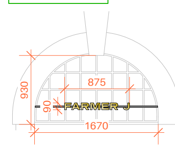
6 Brass Lettering Scale: 1:50
