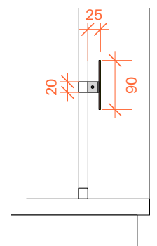
6a Brass Lettering Section Scale: 1:10
