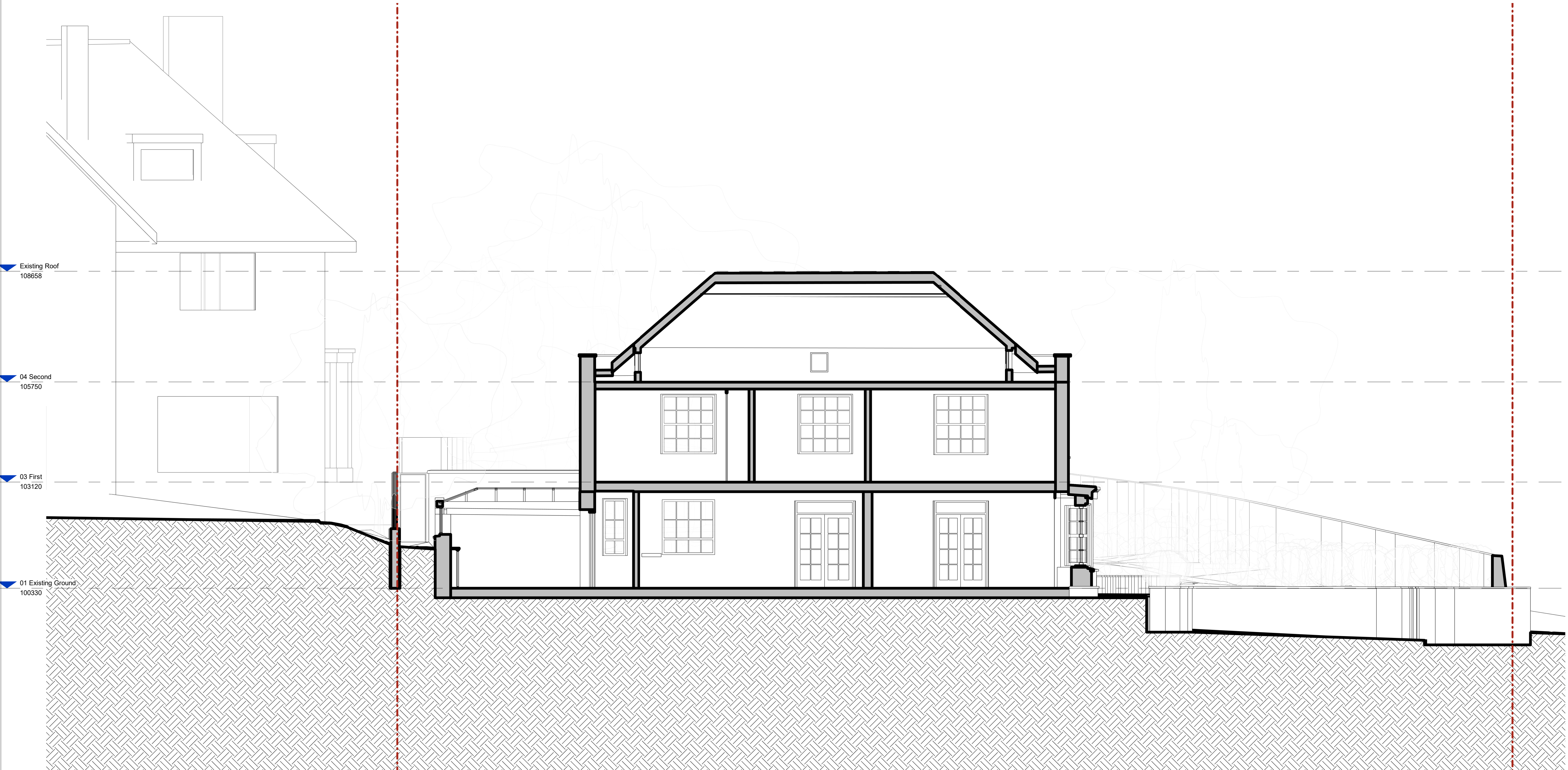
1 Existing Section 2 1 : 50
