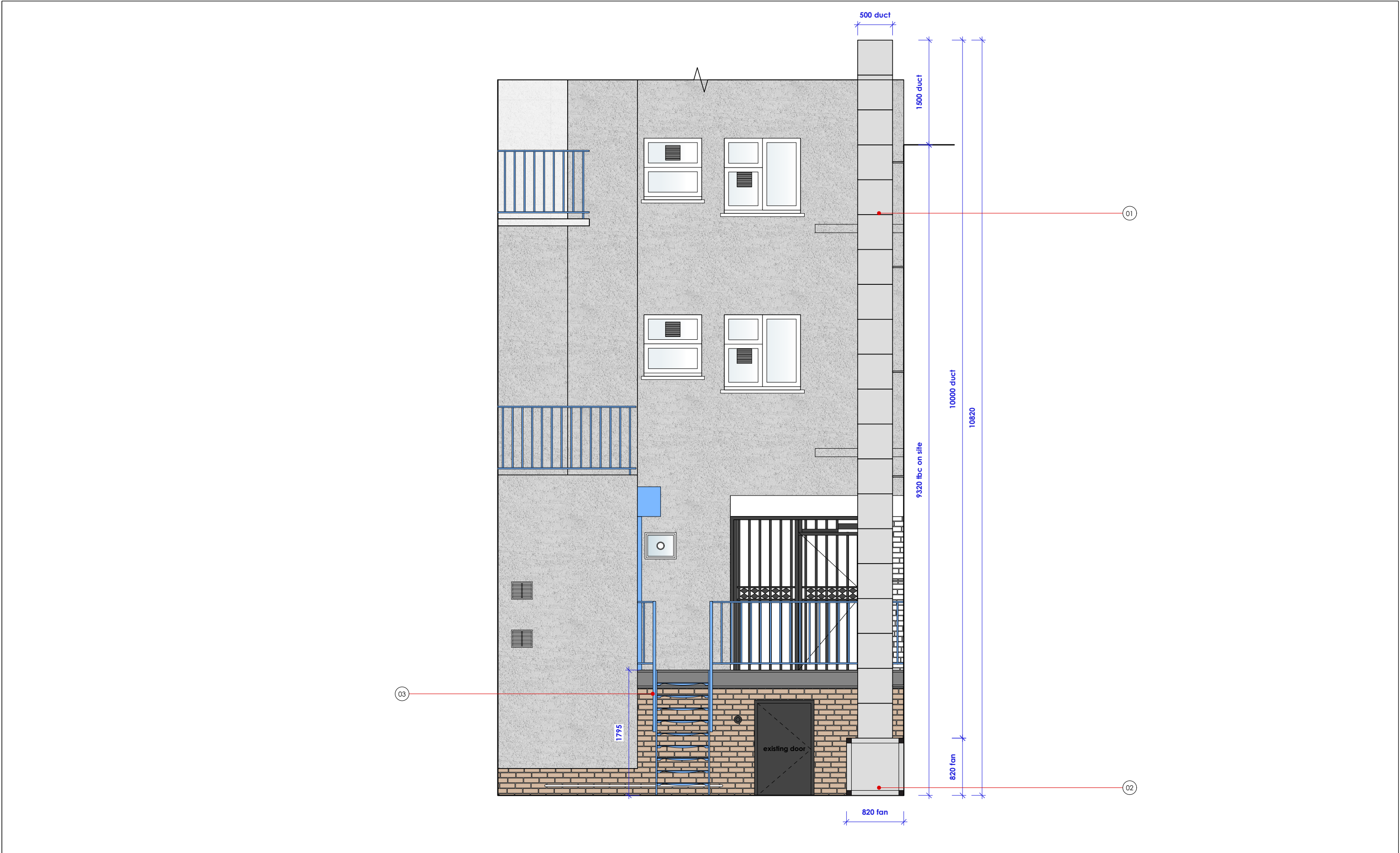
ELEVATION BB
