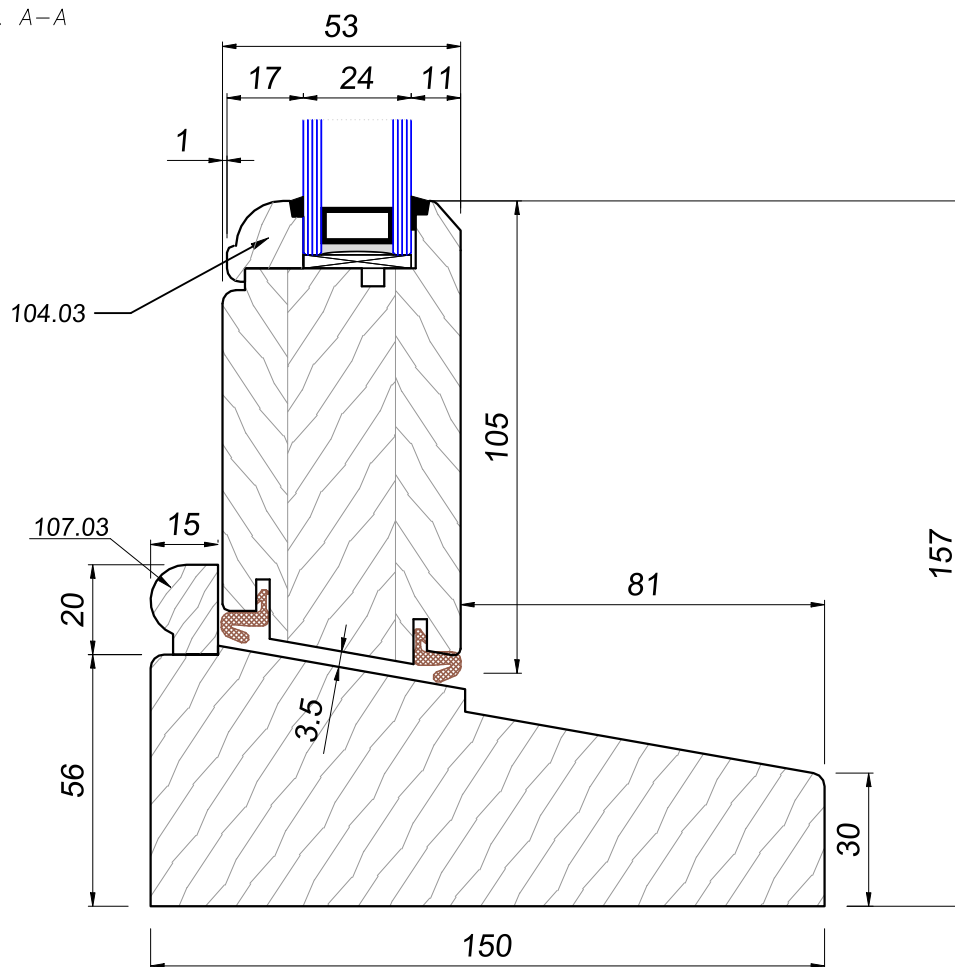
Przek. A-A
