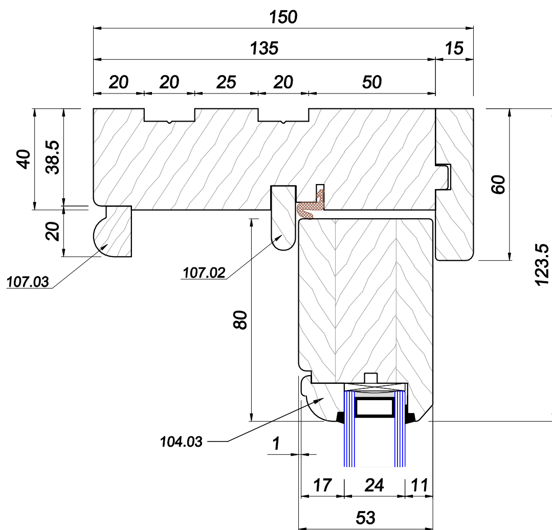
Przek. A-A
