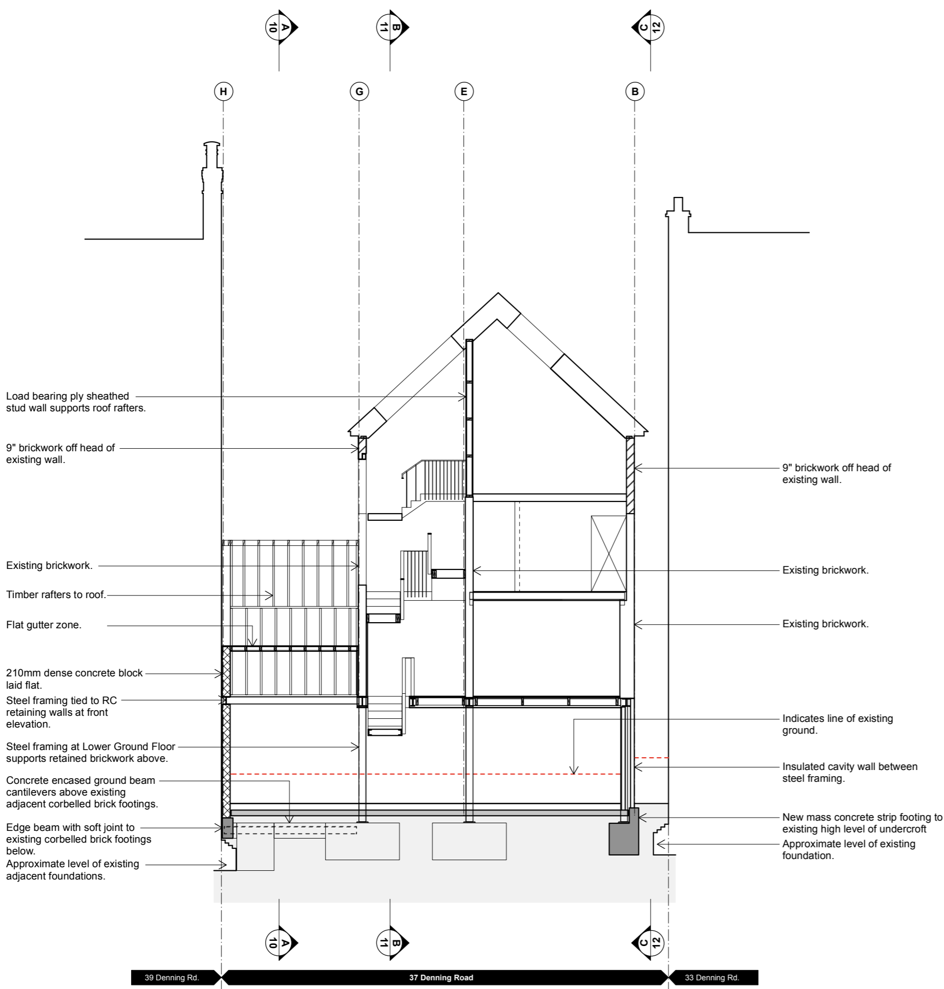
14_Section E.E
