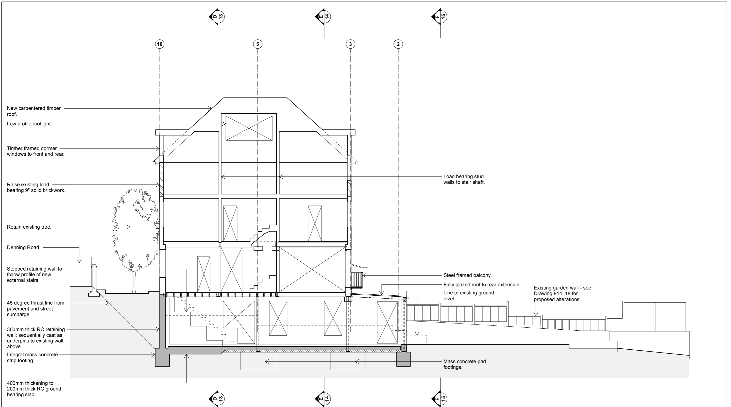
11_Section B.B
