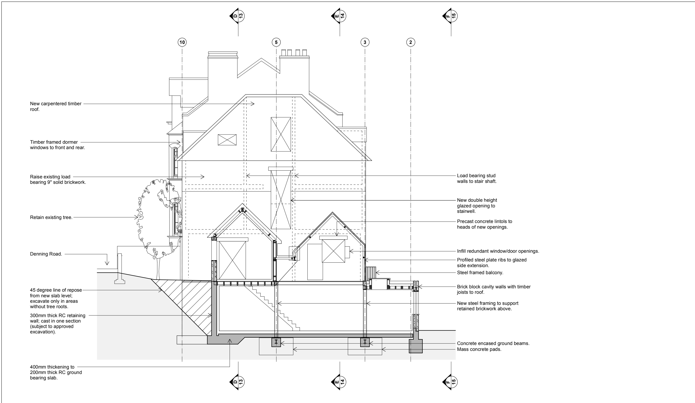
10_Section A.A
