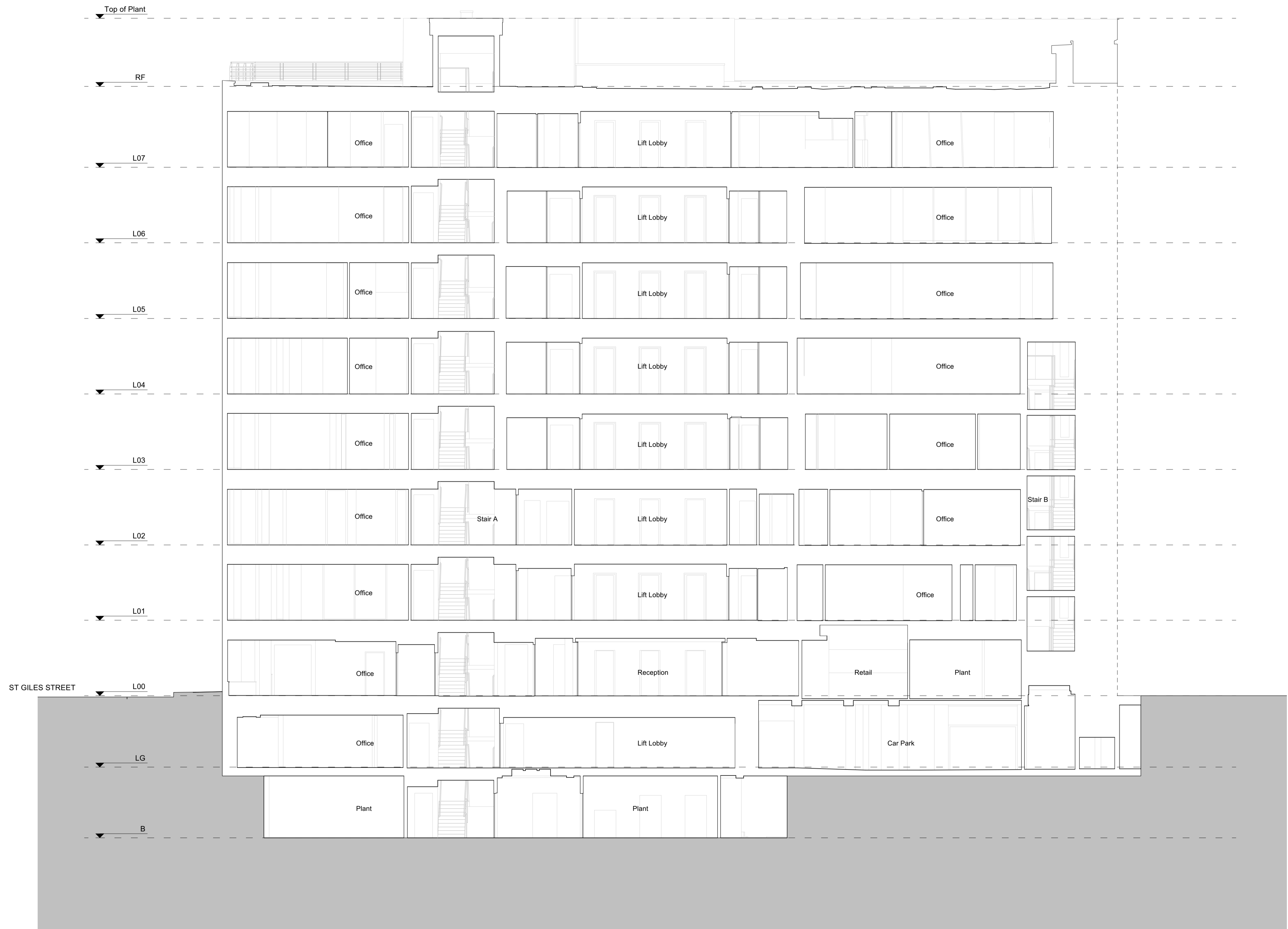
1 Existing Section BB Scale: 1:100
