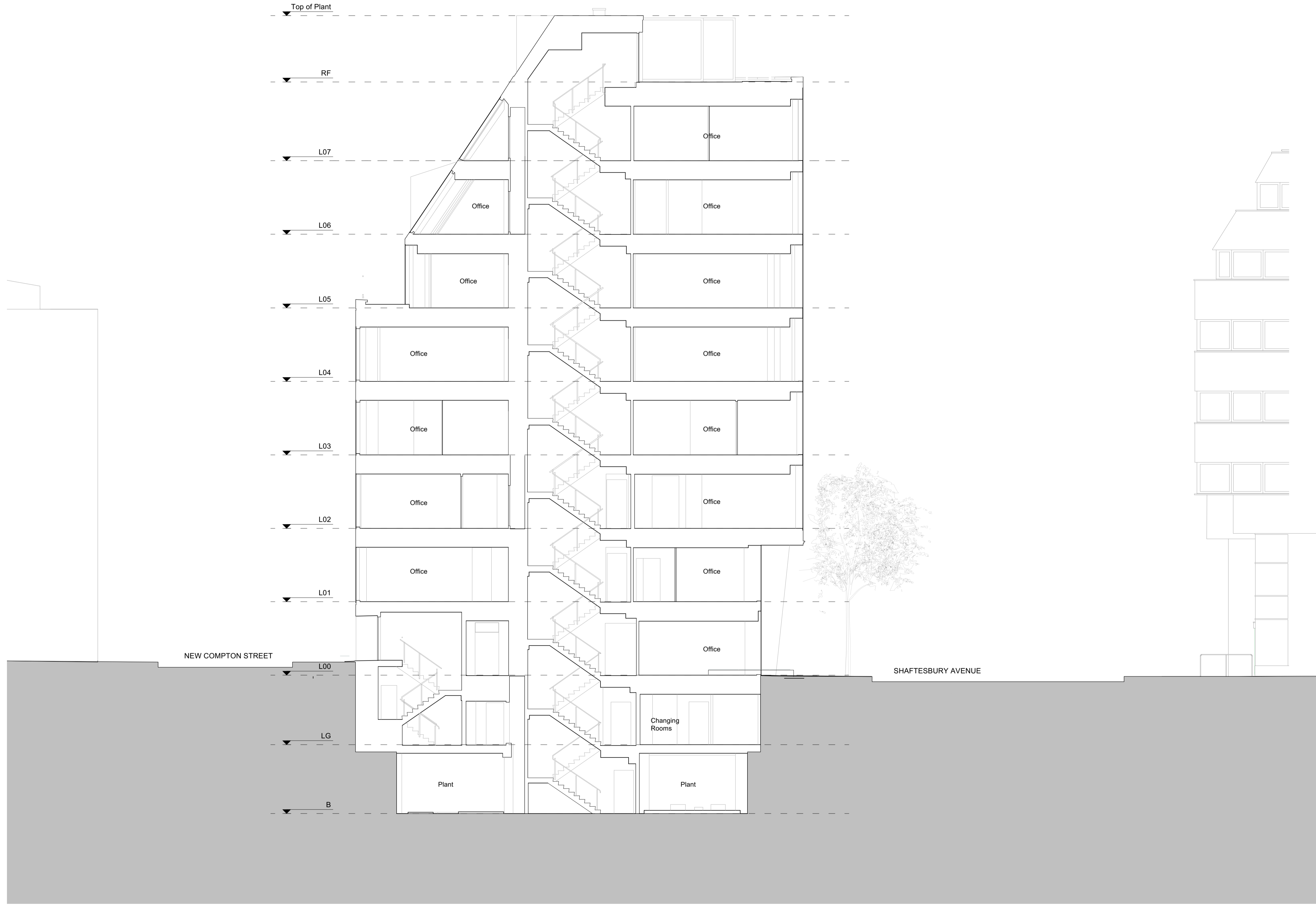
1 Existing Section AA Scale: 1:100
