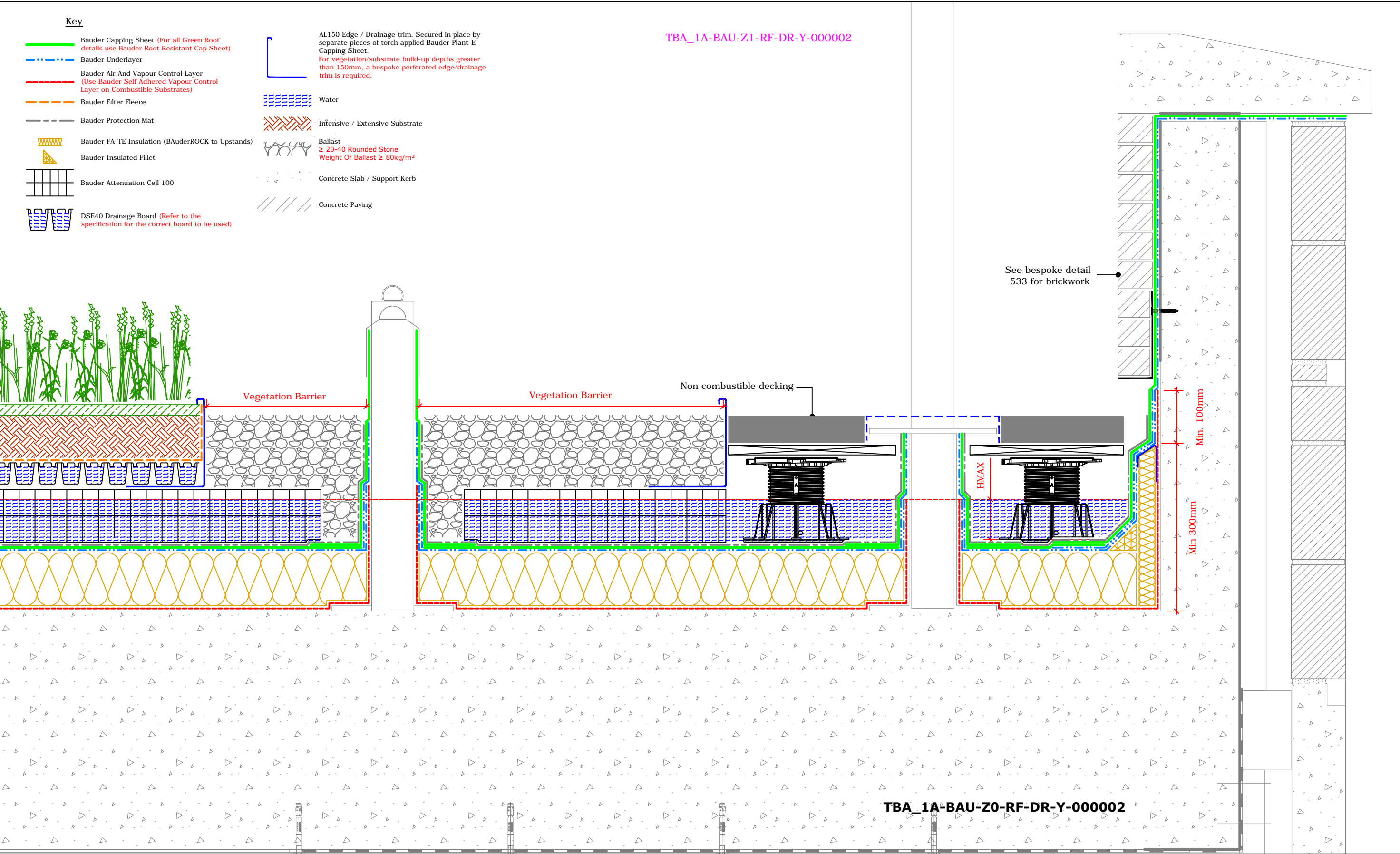
Bespoke Detail - 205 & 20 - 202 & 20 203 & 20 204 & 421 & 423 & 553 & 554 & 555
