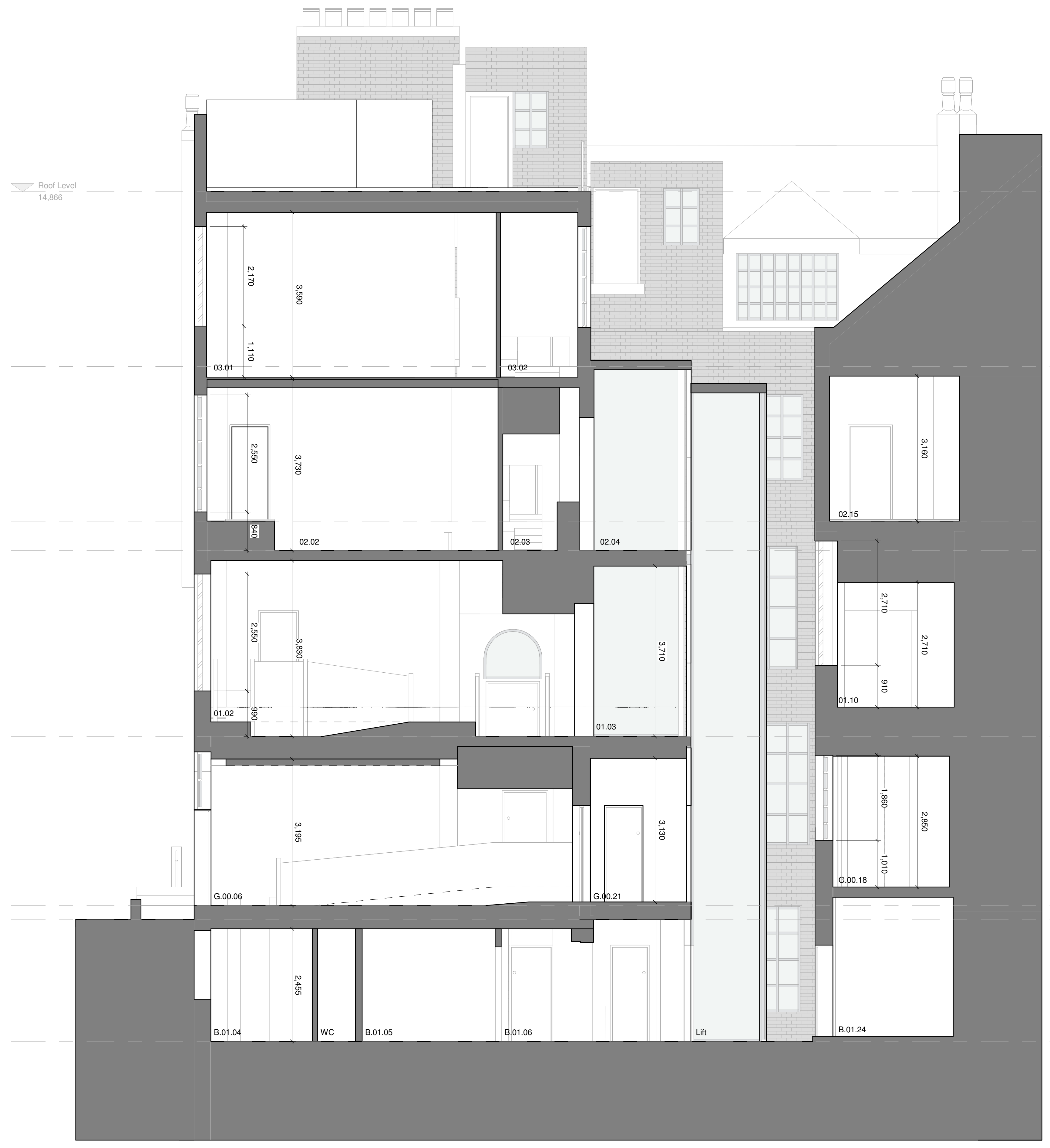
Existing Section C - C 1 : 50
