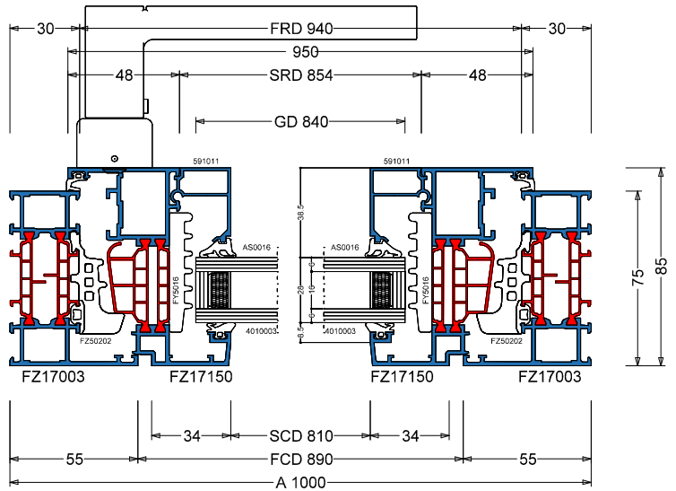
Cross section 3 A - A (Scale: 1:1)
