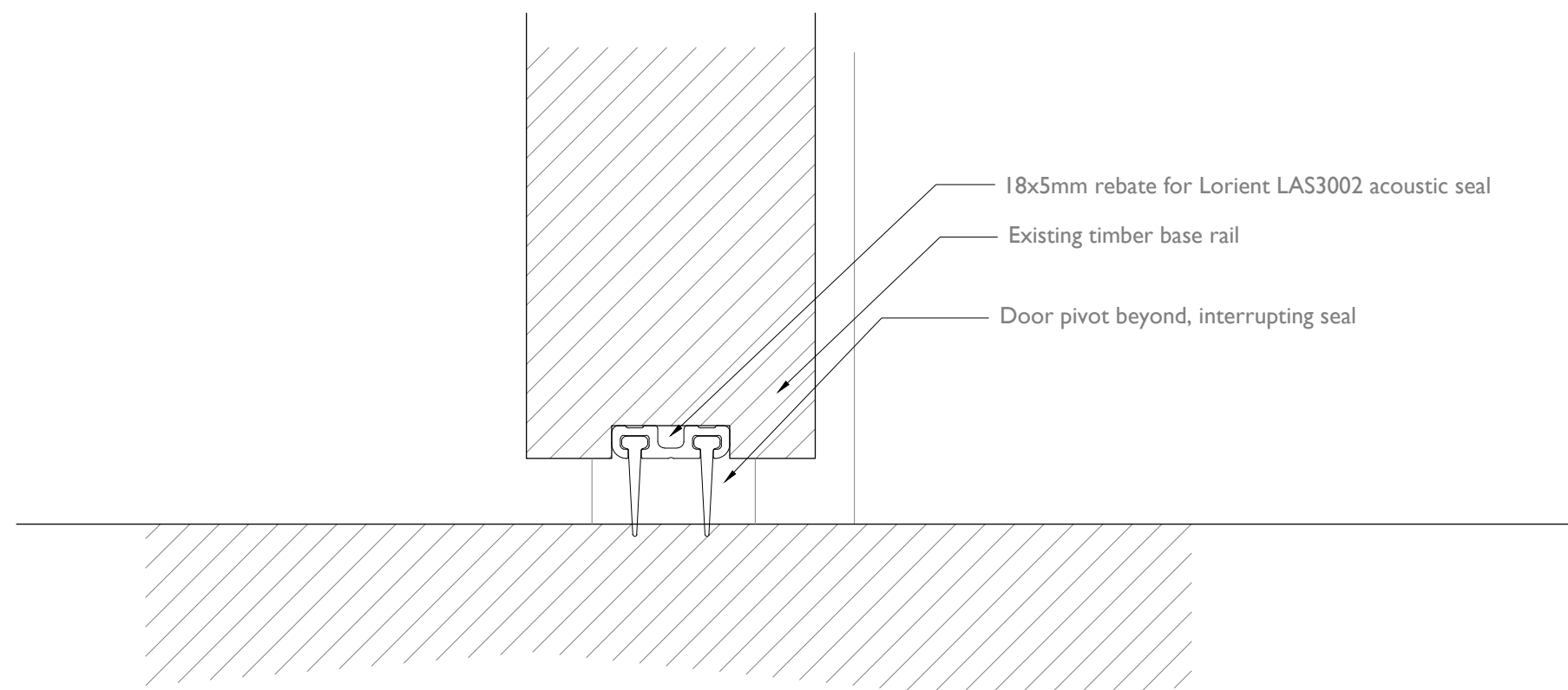
5 DOOR BASE DETAIL 1:1
