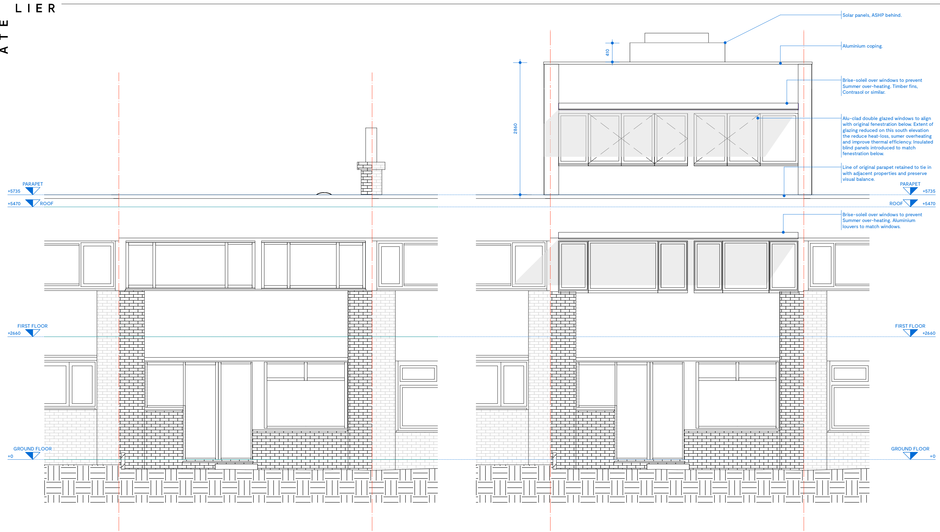
1 EXISTING | REAR ELEVATION SCALE: 1:50
