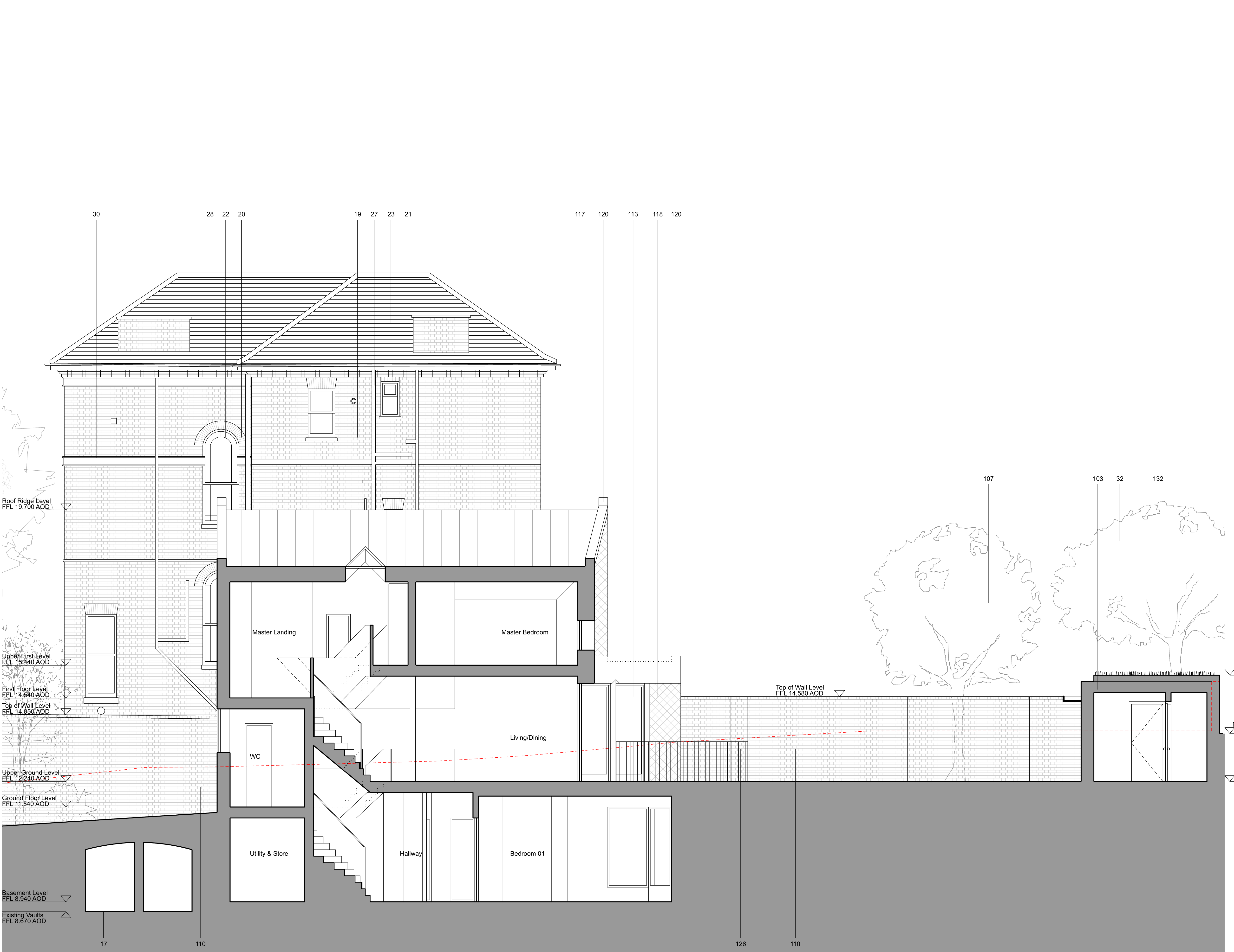
01 - SECTION BB
